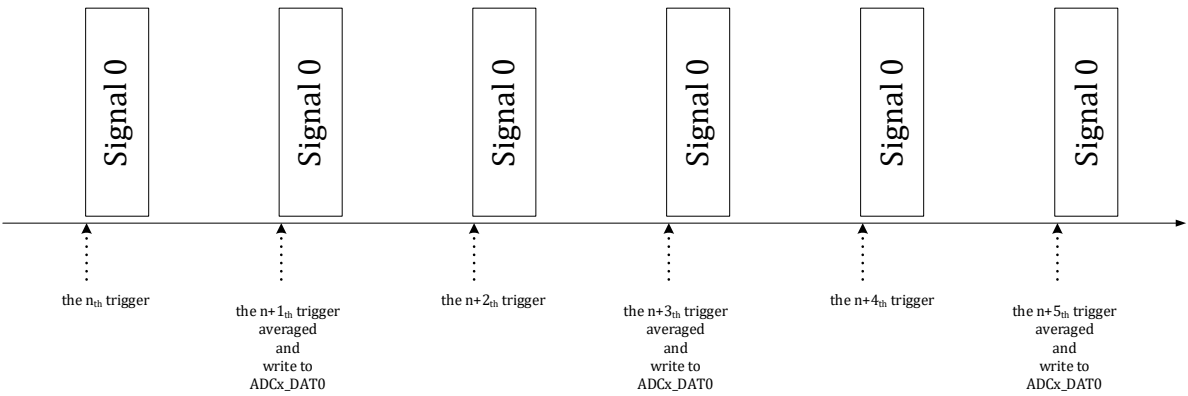
图 13-3 过采样转换时序示例 1
