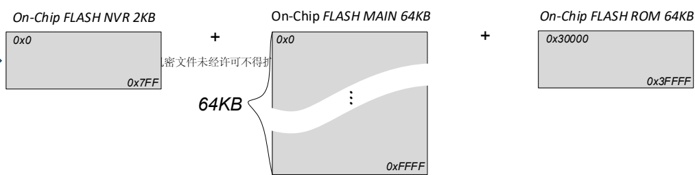
NVR 2KB/MAIN 64KB
