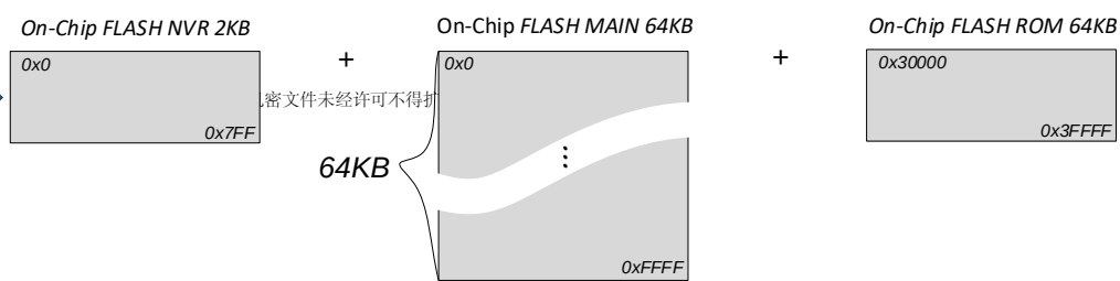
NVR 2KB/MAIN 64KB
