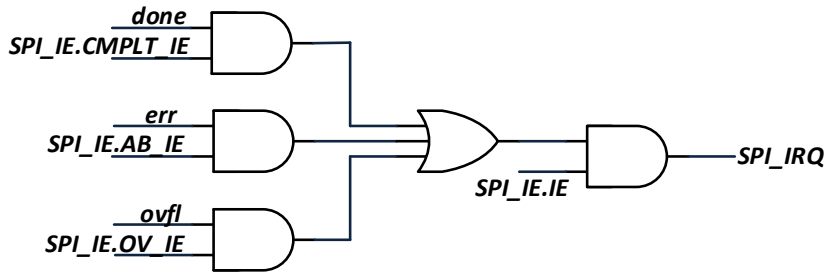
图 19-6 SPI 模块中断选信号产生图
