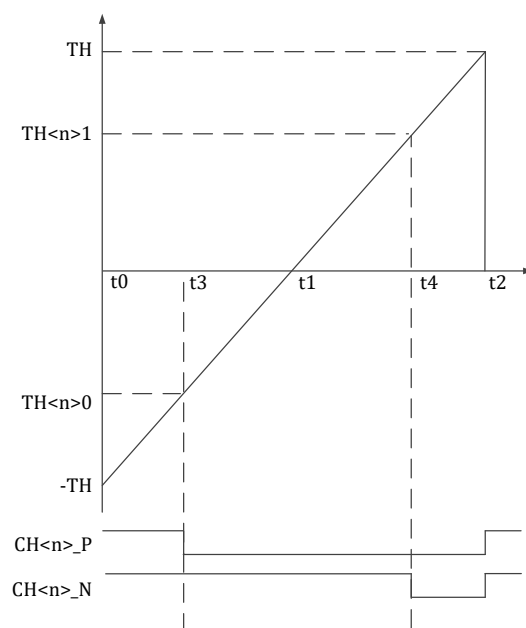
图 16-12 MCPWM 时序边沿对齐模式
