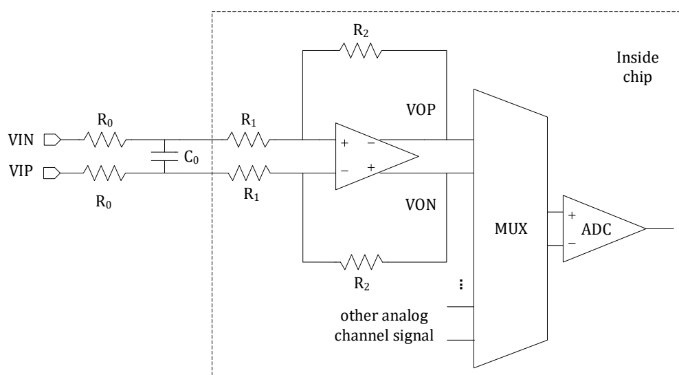
图 5-2 放大器框图
