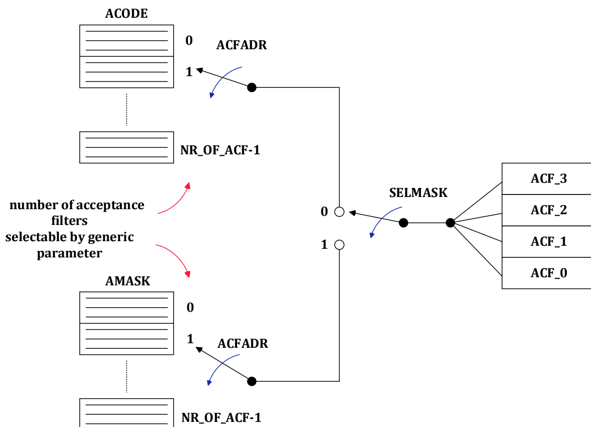
图 21-7 接收过滤器
