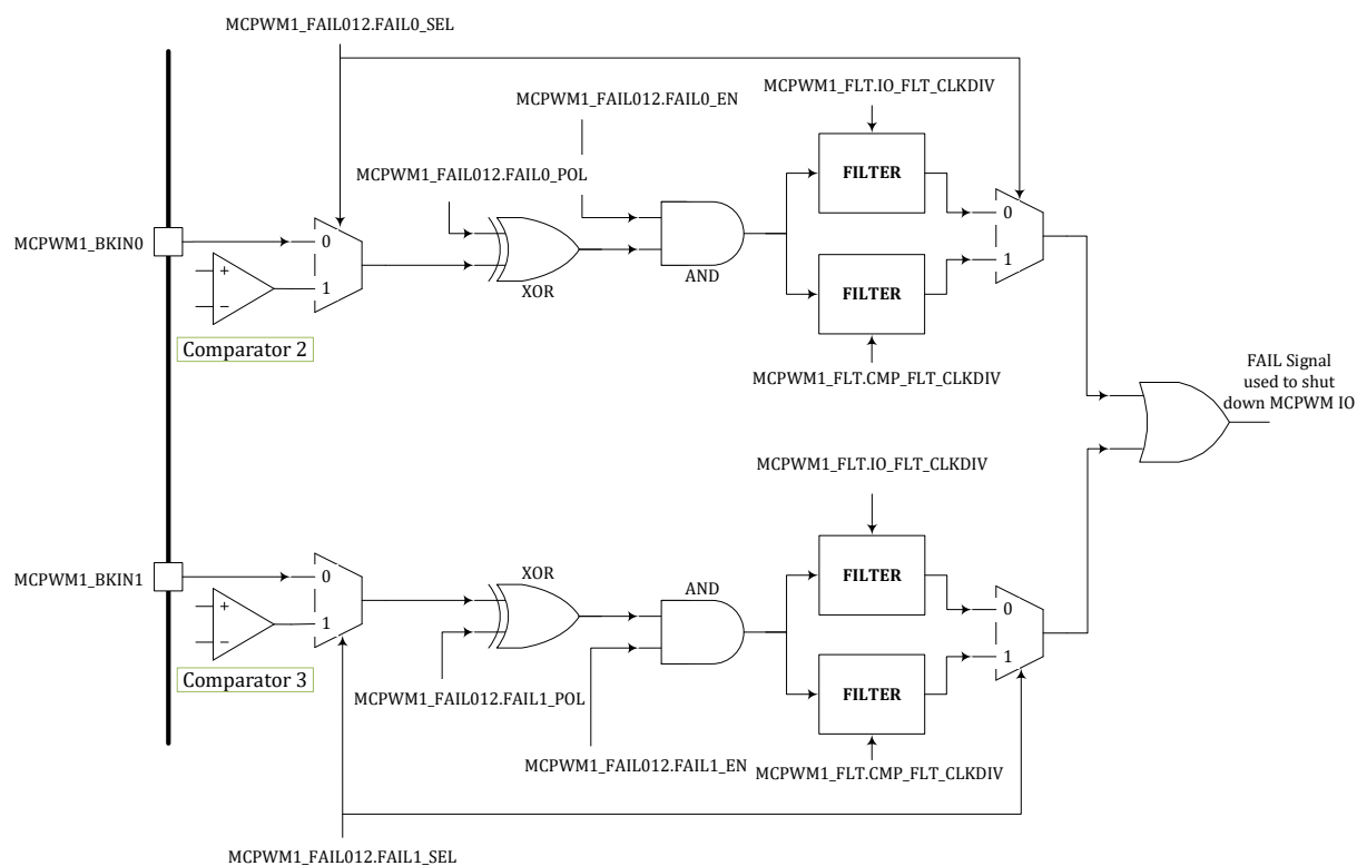
图 16-6 MCPWM1 FAIL0/1 逻辑示意图
