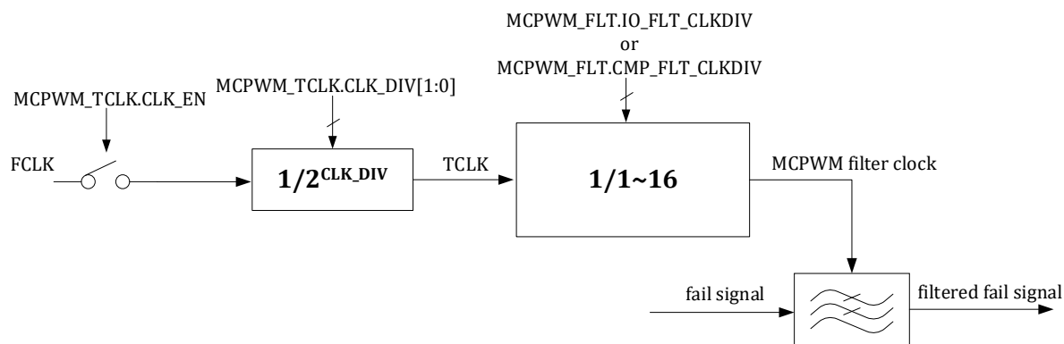
图 16-8 MCPWM Fail 信号滤波时钟生成逻辑
