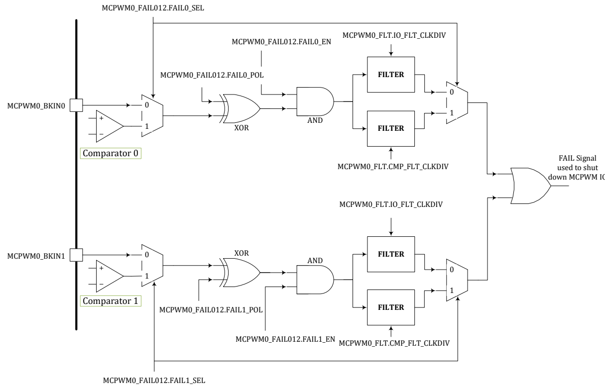
图 16-4 MCPWM0 FAIL0/1 逻辑示意图
