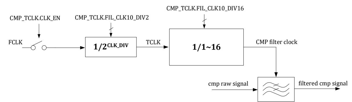
图 20-1 比较器滤波时钟产生
