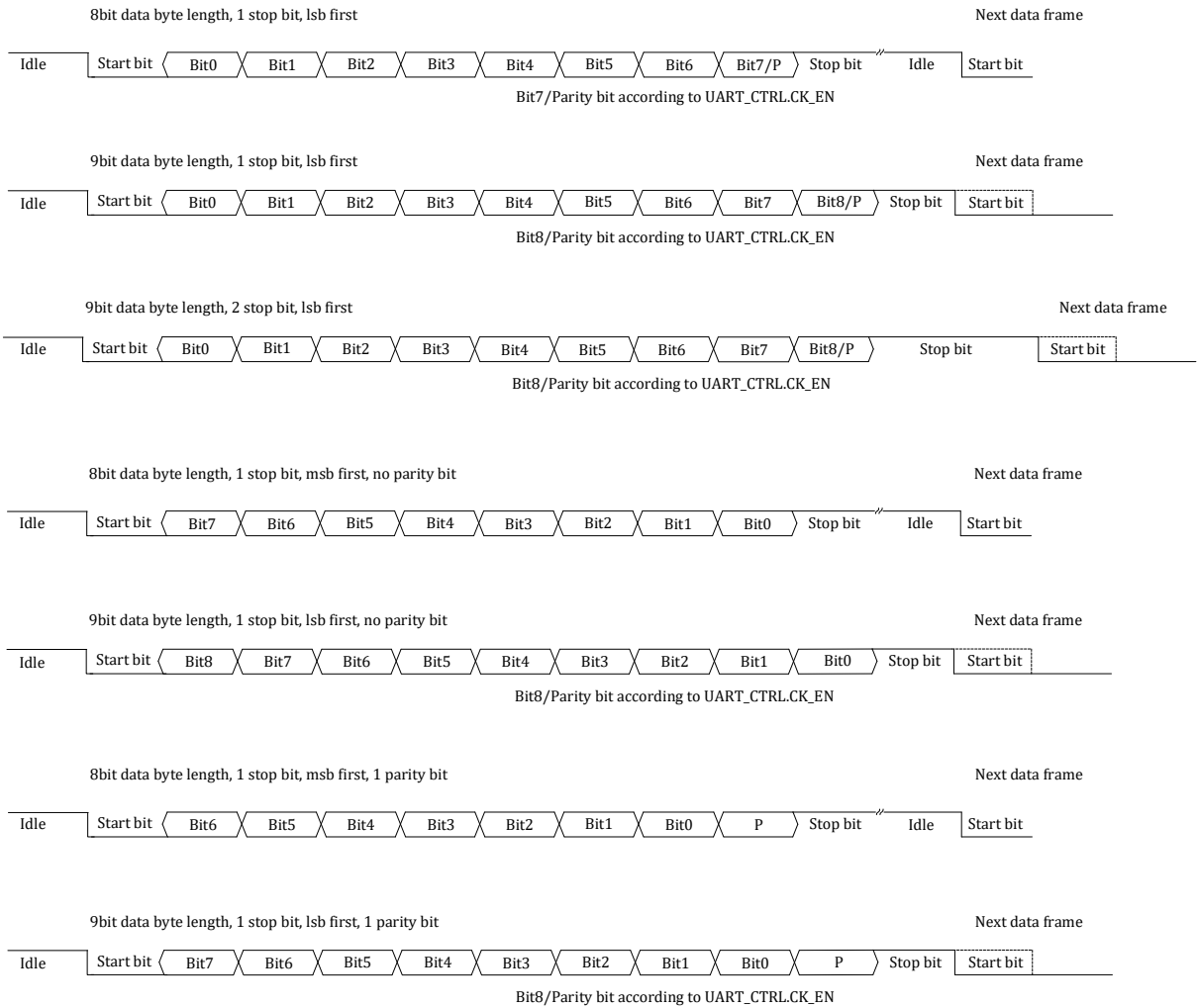
图 17-1 UART 帧格式
