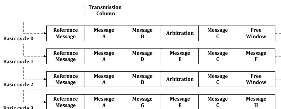
图 21-12 TTCAN 时空矩阵示例
