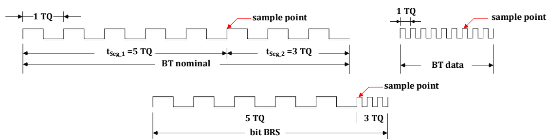
图 21-15 比特 BRS 的波特率切换 S\_PRESC \neq F\_PRESC
