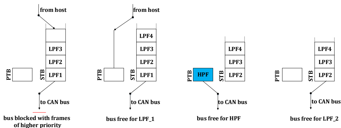
图 21-3 发送缓冲器应用示例 (TSALL=1)
