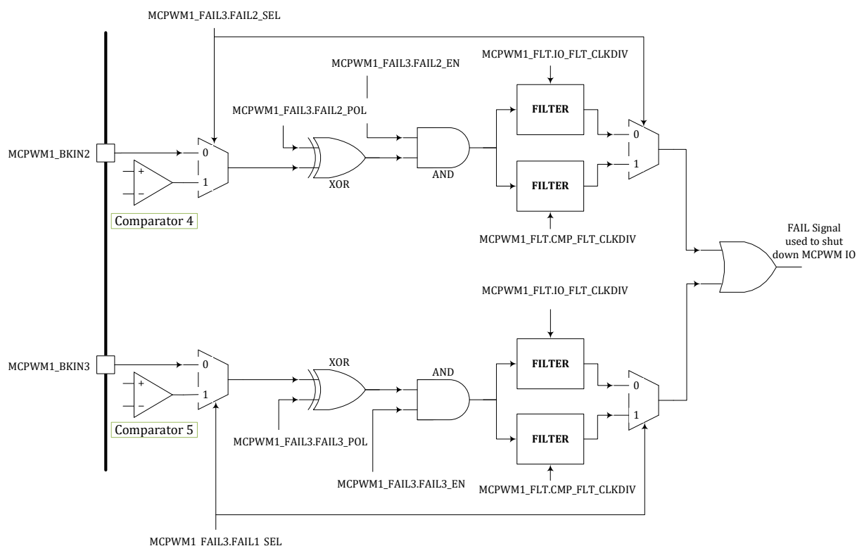
图 16-7 MCPWM1 FAIL2/3 逻辑示意图
