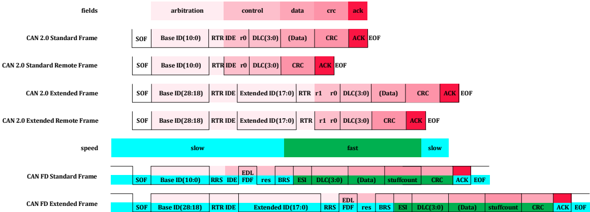
图 21-4 CAN 2.0 和 CAN FD 帧类型
