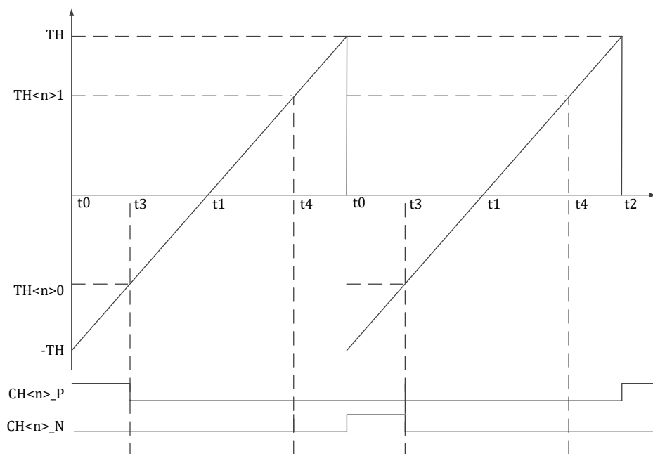
图 16-13 MCPWM 时序 TH&lt;n&gt;0 和 TH&lt;n&gt;1 边沿对齐推挽模式
