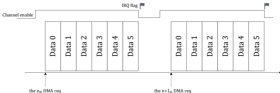
图 8-6 CIRC=1 且 RMODE=0 DMA 传输情况
