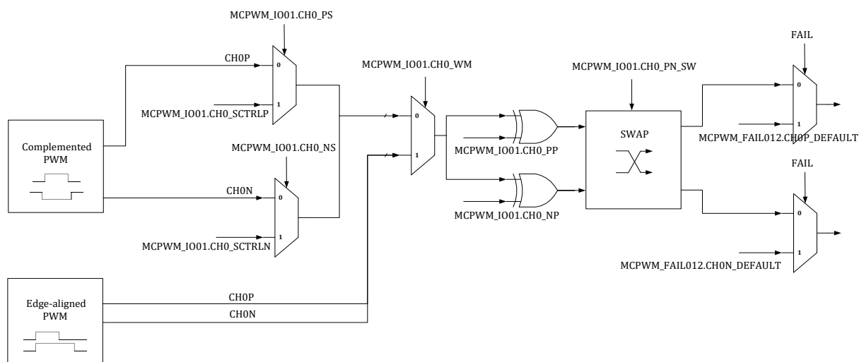
图 16-9 IO Driver 模块数据流程图
