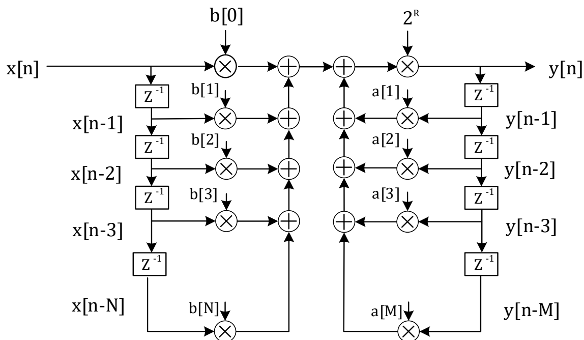
图 12-9 直接 1 型 IIR 滤波器结构
