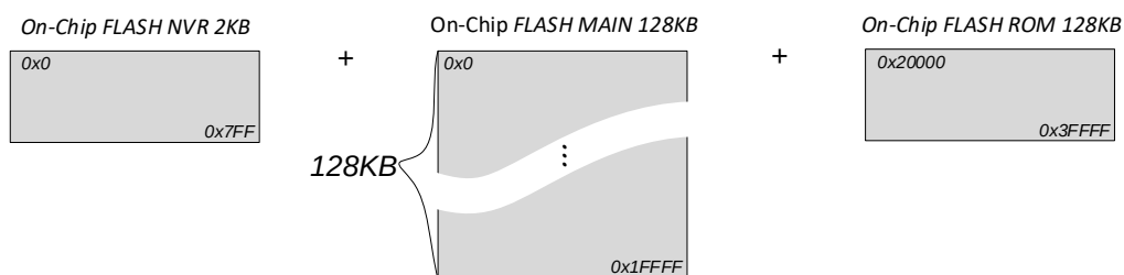
NVR 2KB/MAIN 128KB
