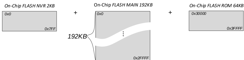
NVR 2KB/MAIN 192KB/ROM 0KB
