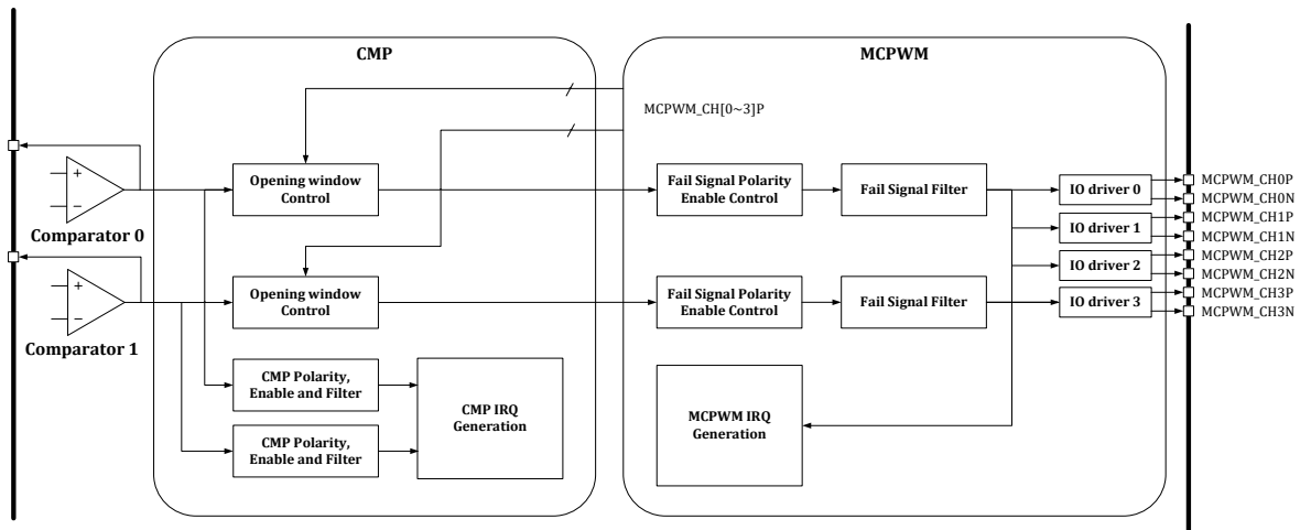
图 20-3 CMP 与 MCPWM 的联动
