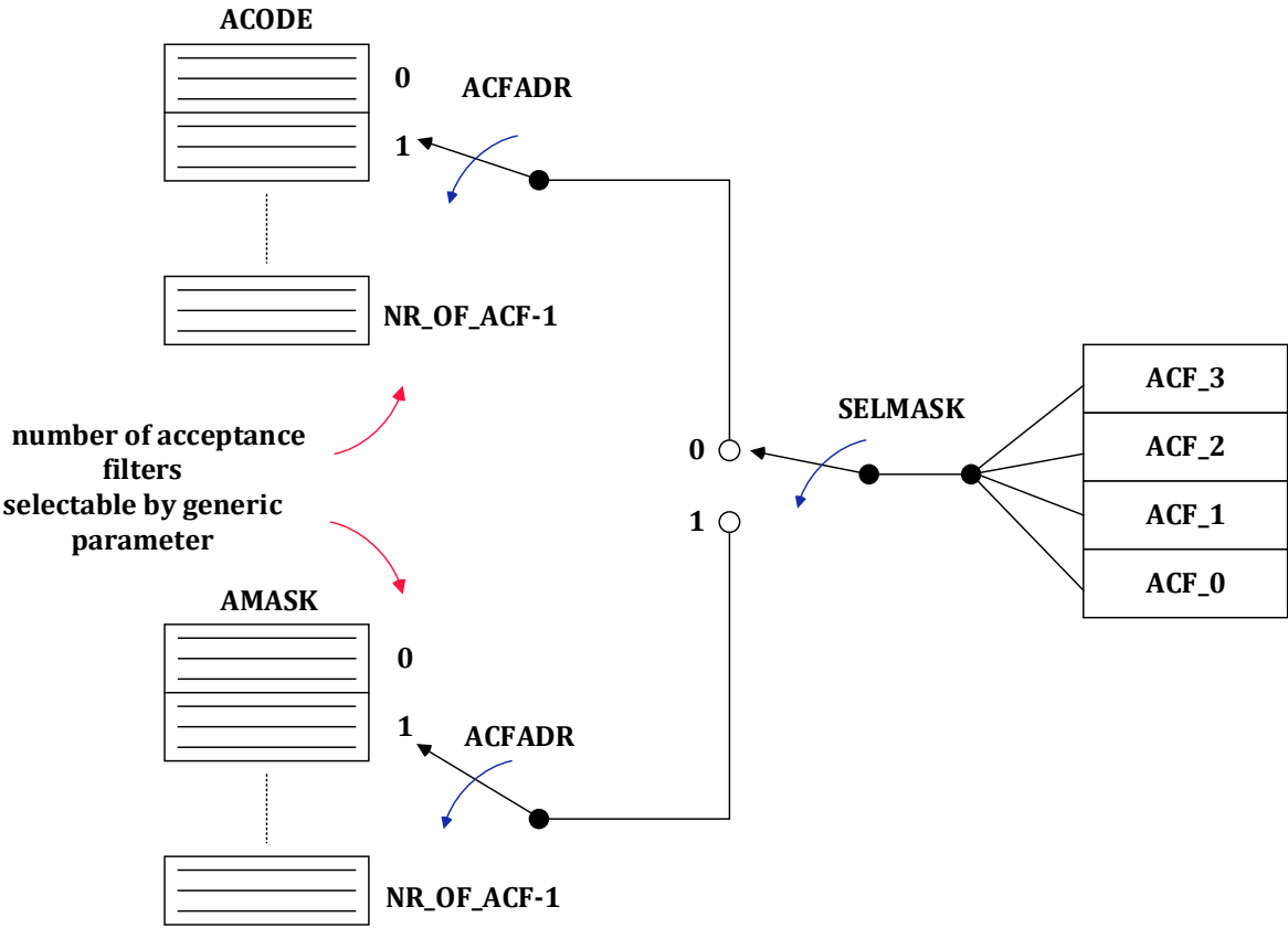
图 21-7 接收过滤器
