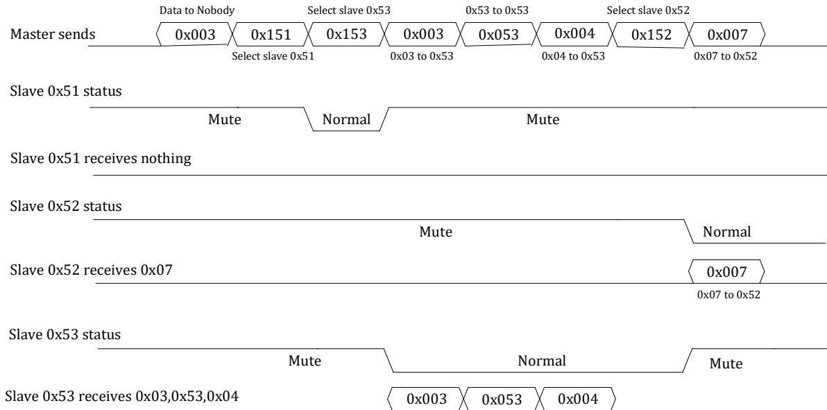
图 17-3 UART 多机通讯示例
