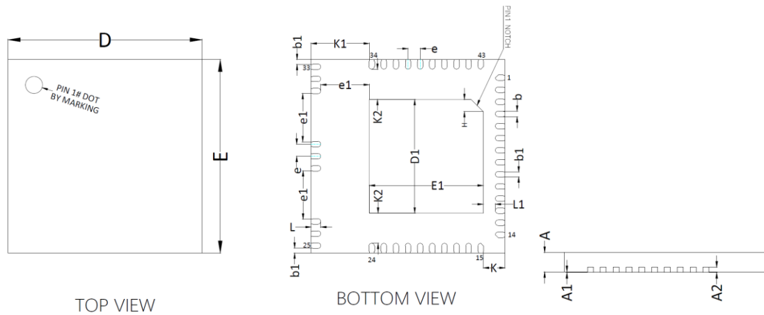
图 4-3 LKS32MC088K22U8Q8 封装图示
