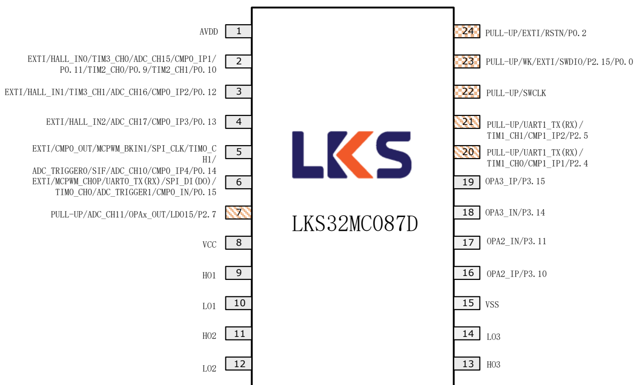
图 3-1 LKS32MC087DM6S8(B)管脚分布图
