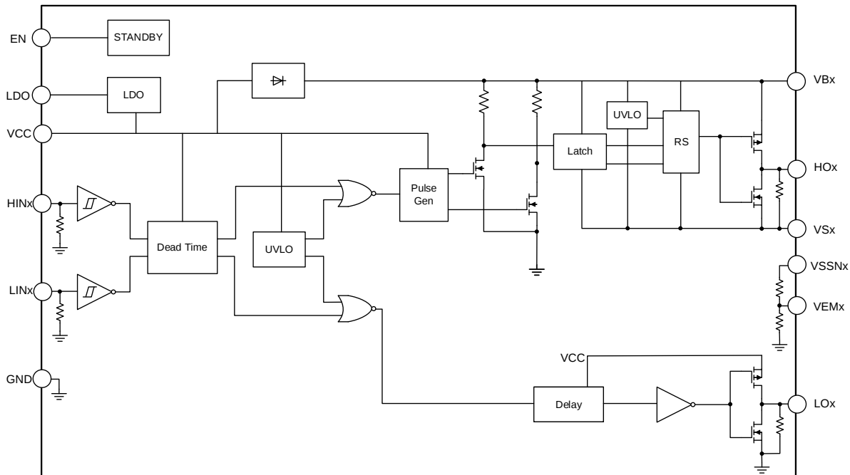
图 22-3 栅极驱动模块 G6 内部框图
