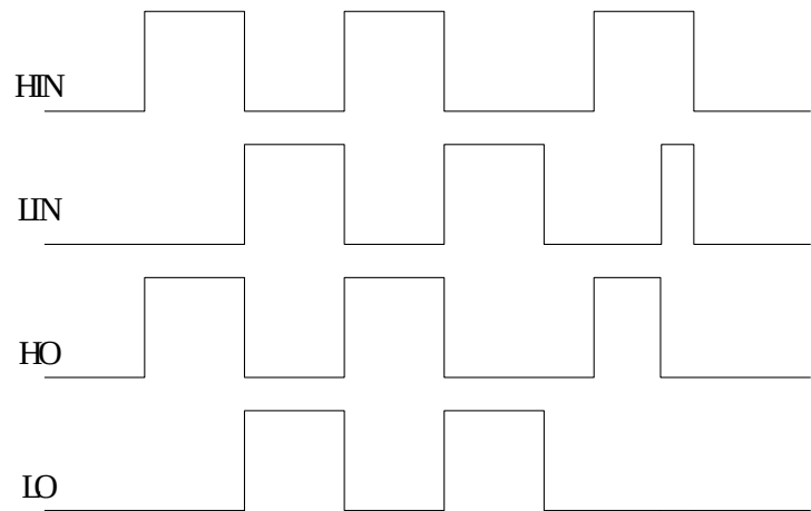
图 22-4 栅极驱动模块 G1/G2/G3/G6 极性示意图
