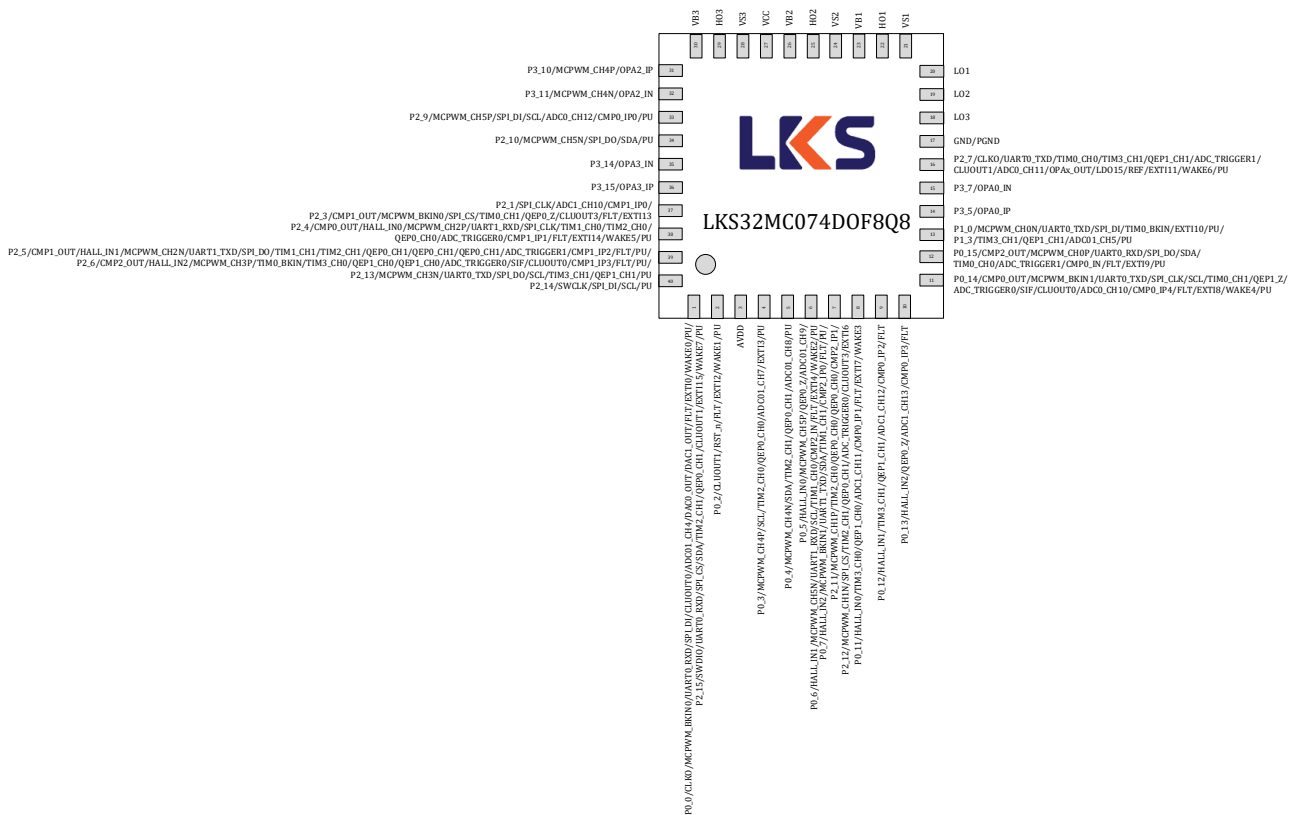
图 3-9 LKS32MC074D0F8Q8 管脚分布图
