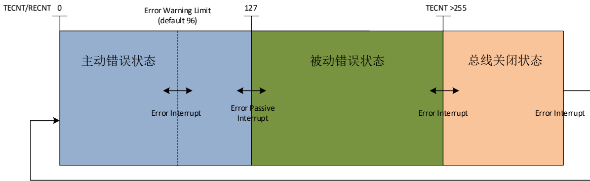
图 24-4 CAN 模块错误管理
