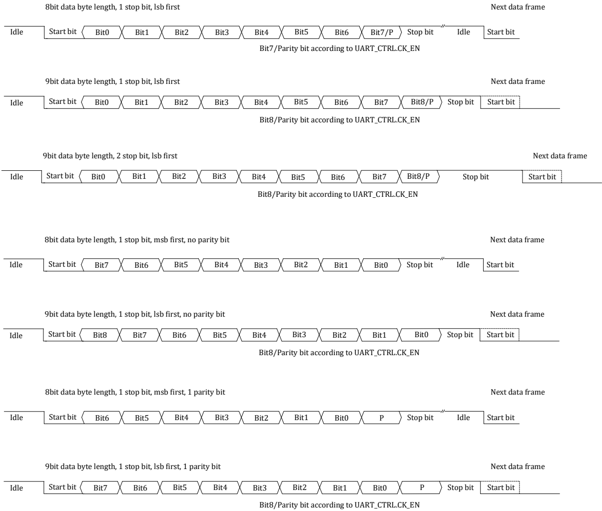
图 17-1 UART 帧格式
