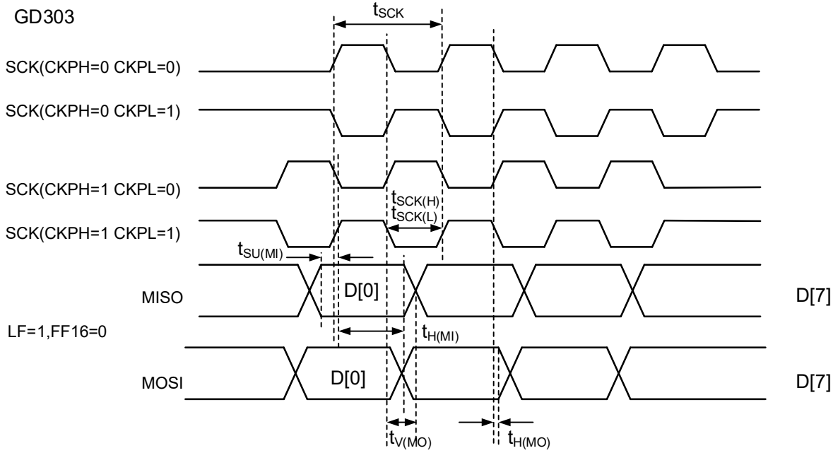
图 11-3 SPI 从机模式
