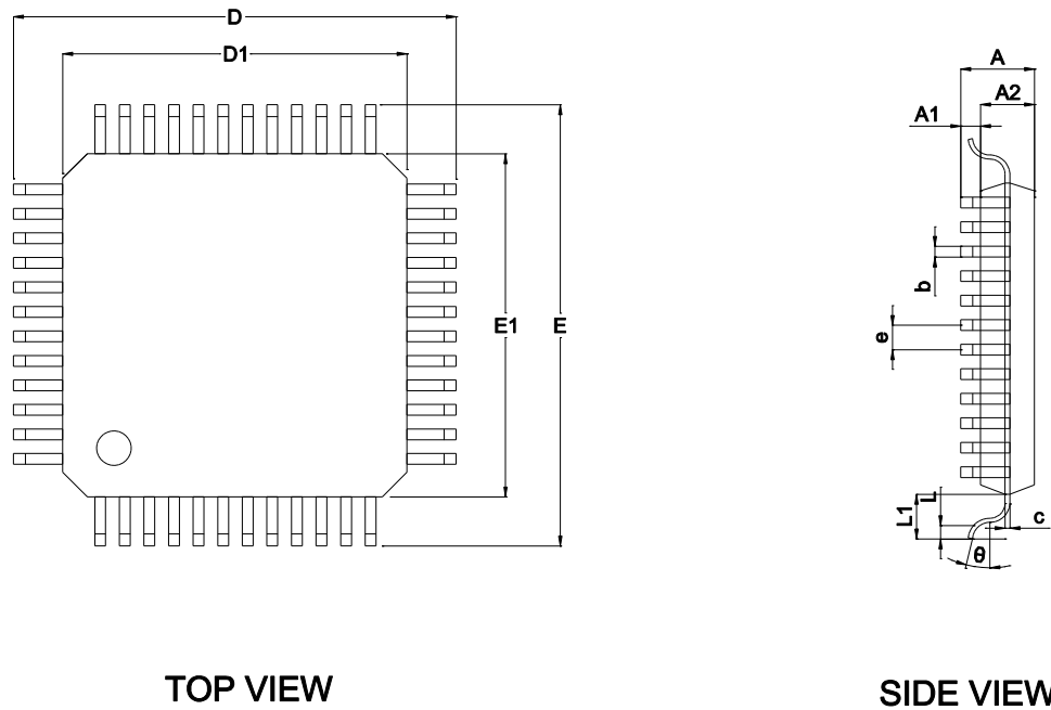
图 4-2 LKS32MC071CBT8/LKS32MC071C8T8 封装图示(TQFP48)
