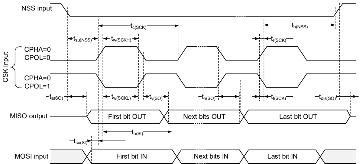
图 11-2 SPI 从机模式且 CHPA=0
