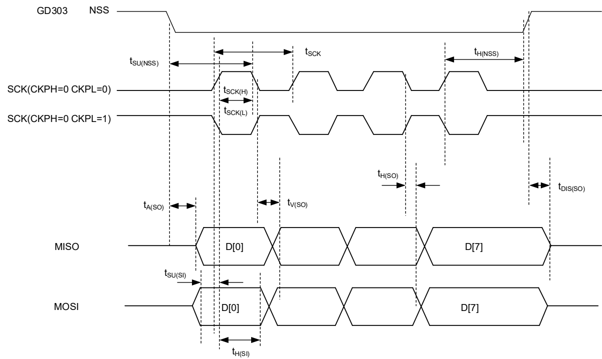
图 11-1 SPI 主机模式
