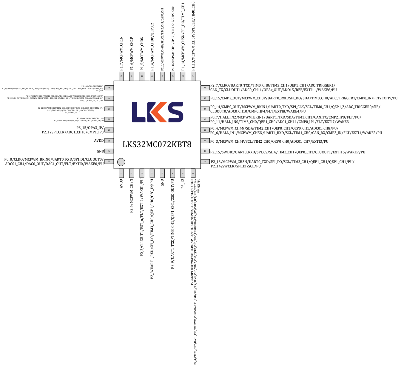
图 3-5 LKS32MC072KBT8 管脚分布图
