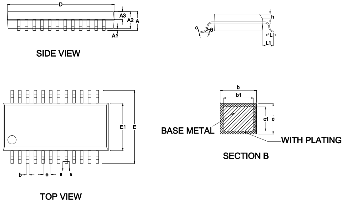
图 4-6 LKS32MC077MBS8 封装图示
