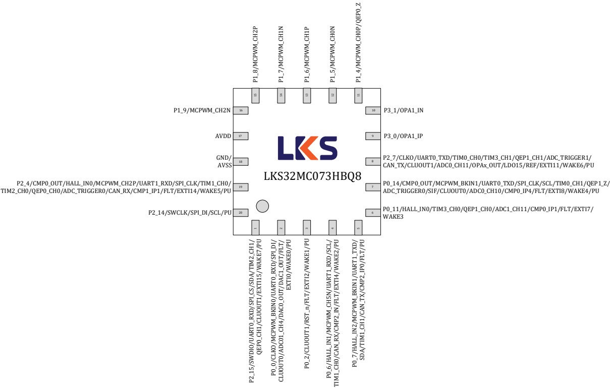
图 3-6 LKS32MC073HBQ8 管脚分布图
