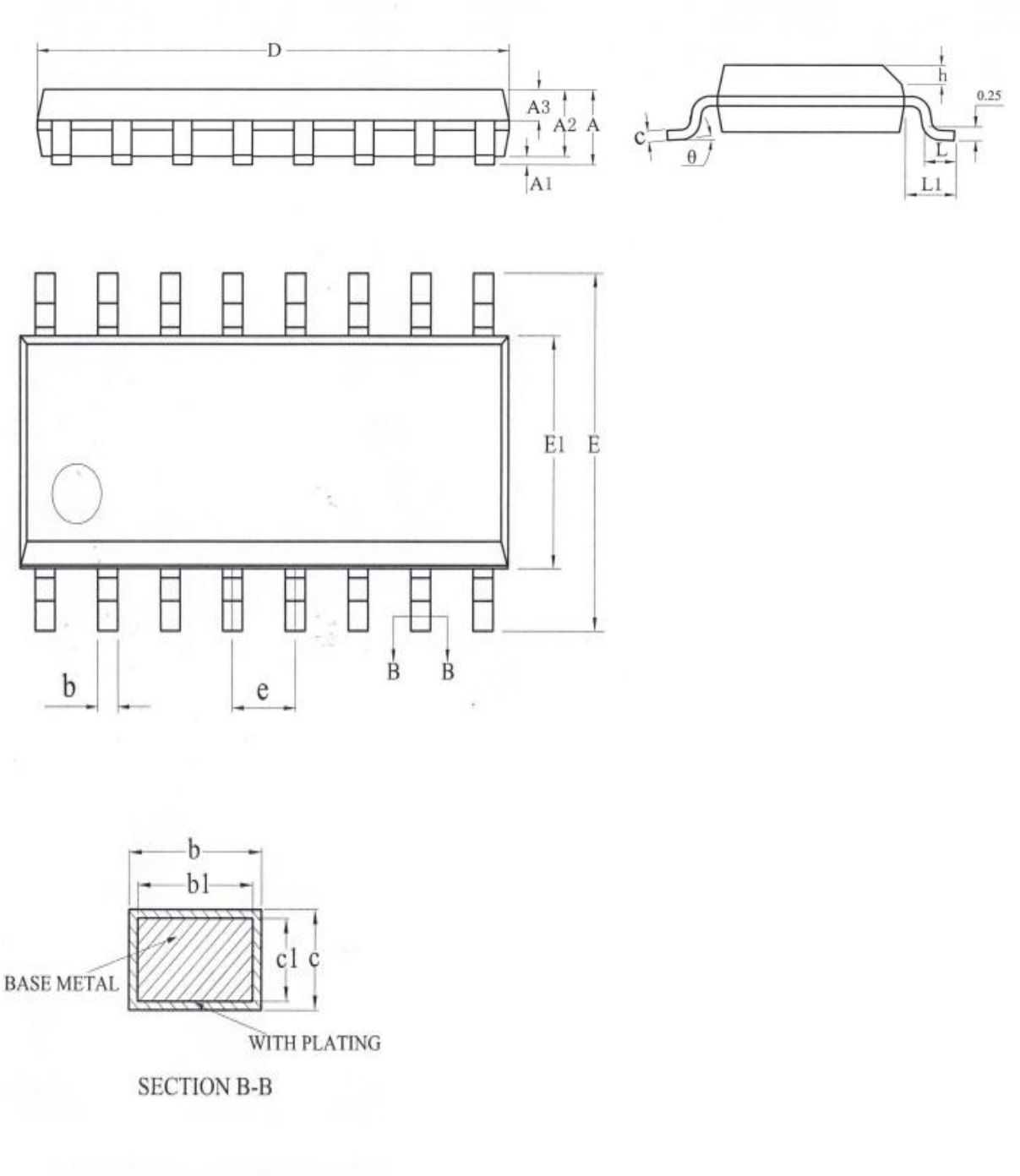
图 4-2 LKS32MC055DL6S8 封装图示
