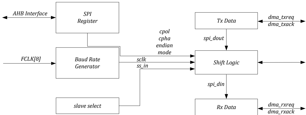
图 8-1 SPI 模块结构框图
