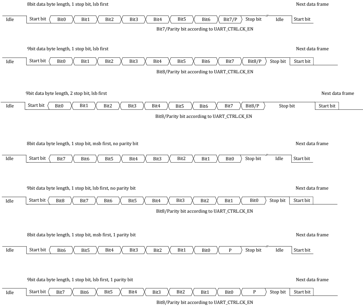
图 16-1 UART 帧格式
