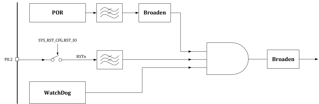
图 6-2 复位架构
