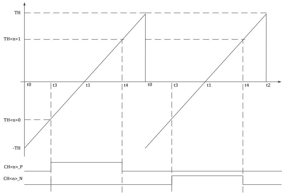
图 14-8 MCPWM 时序 TH<n>0 和 TH<n>1-中心对齐推挽模式
