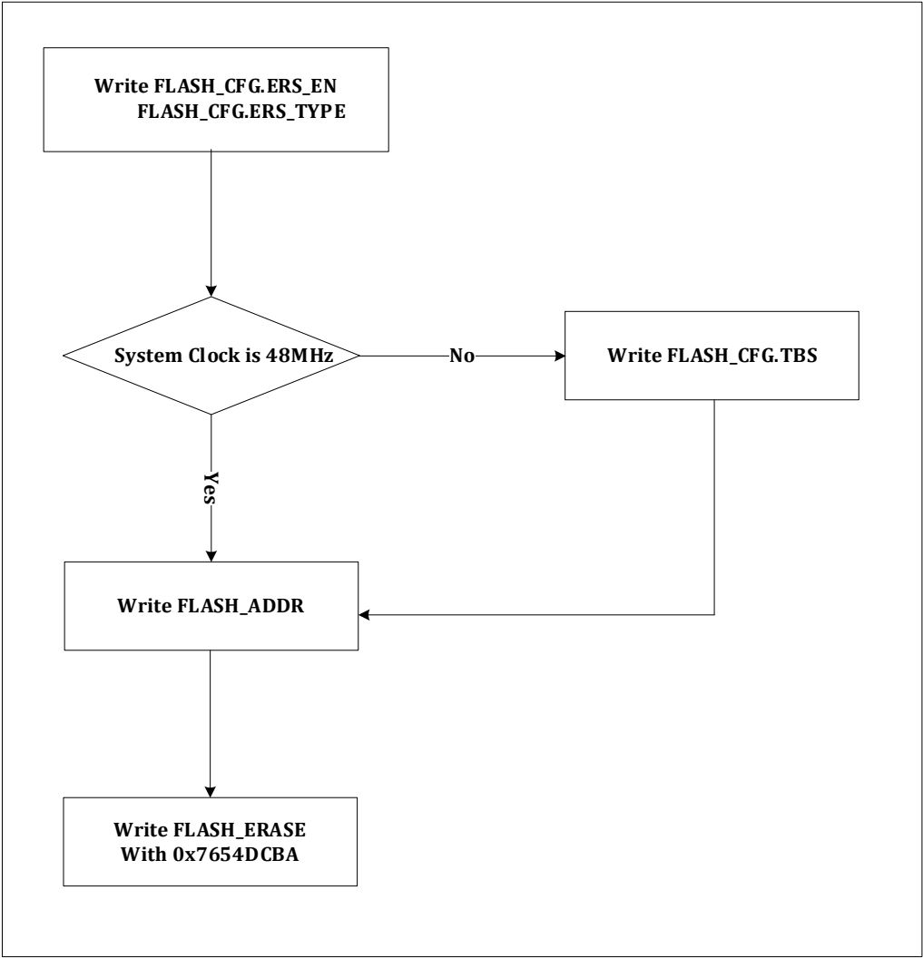
图 7-6 FLASH 模块擦除操作流程
