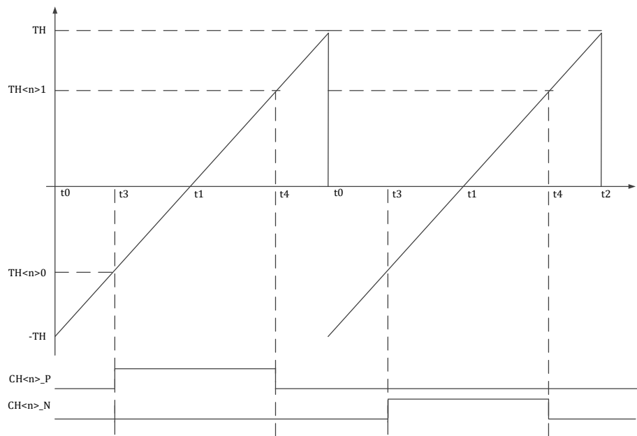
图 14-8 MCPWM 时序 TH\langle n \rangle_0 和 TH\langle n \rangle_1 -中心对齐推挽模式
