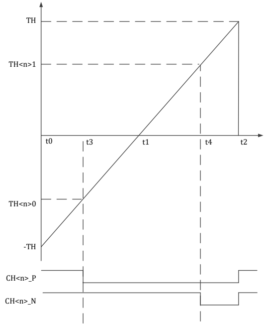
图 14-9MCPWM 时序边沿对齐模式
