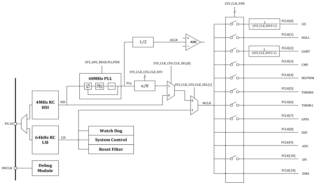
图 6-1 时钟架构
