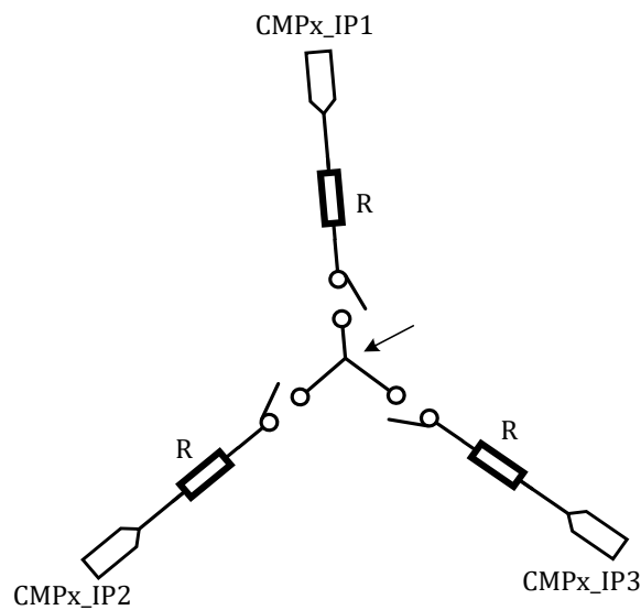
图 5-5 BEMFx_MID 信号
