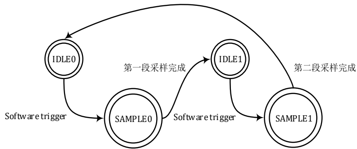
图 12-4 ADC 两段采样状态转移图
