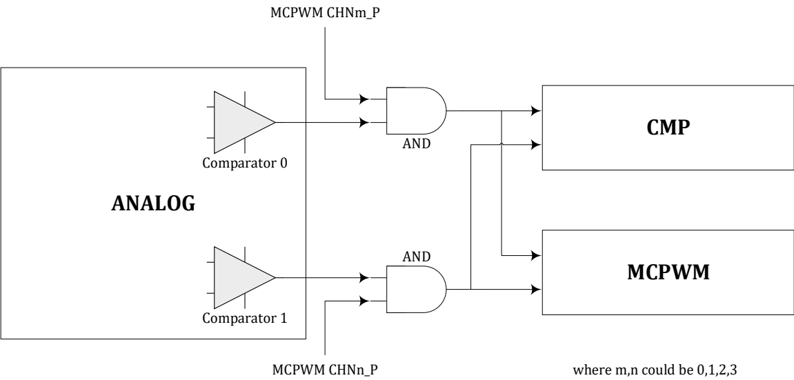
图 10-4 比较器开窗功能图示
