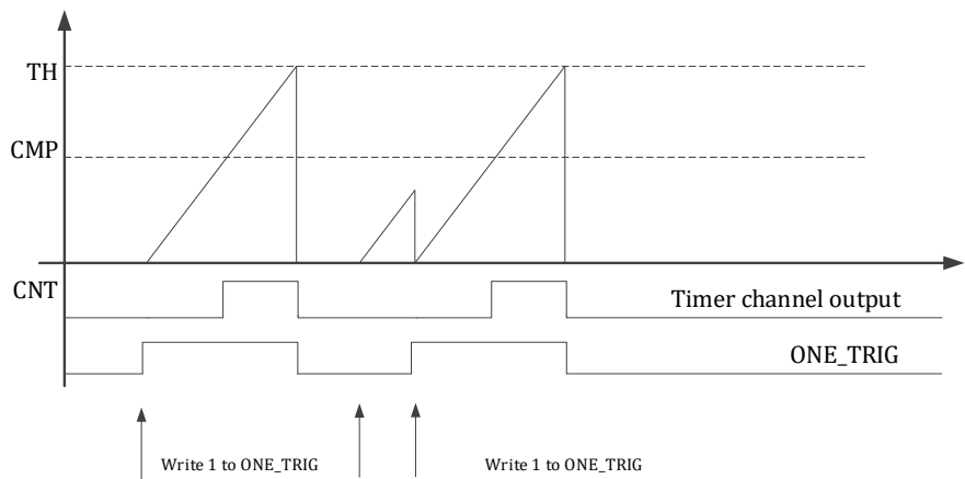
图 13-6 UTimer 单次触发模式
