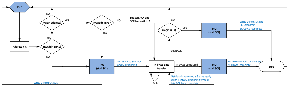
图 9-4 从模式下多字节发送示意图
