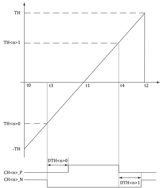
图 14-7MCPWM 时序 TH\langle n \rangle_0 和 TH\langle n \rangle_1 -中心对齐模式
