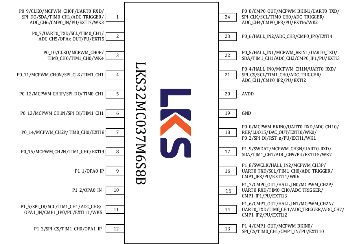
图 3-7 LKS32MC037M6S8B/LKS32MC037M6S8C 管脚分布图
