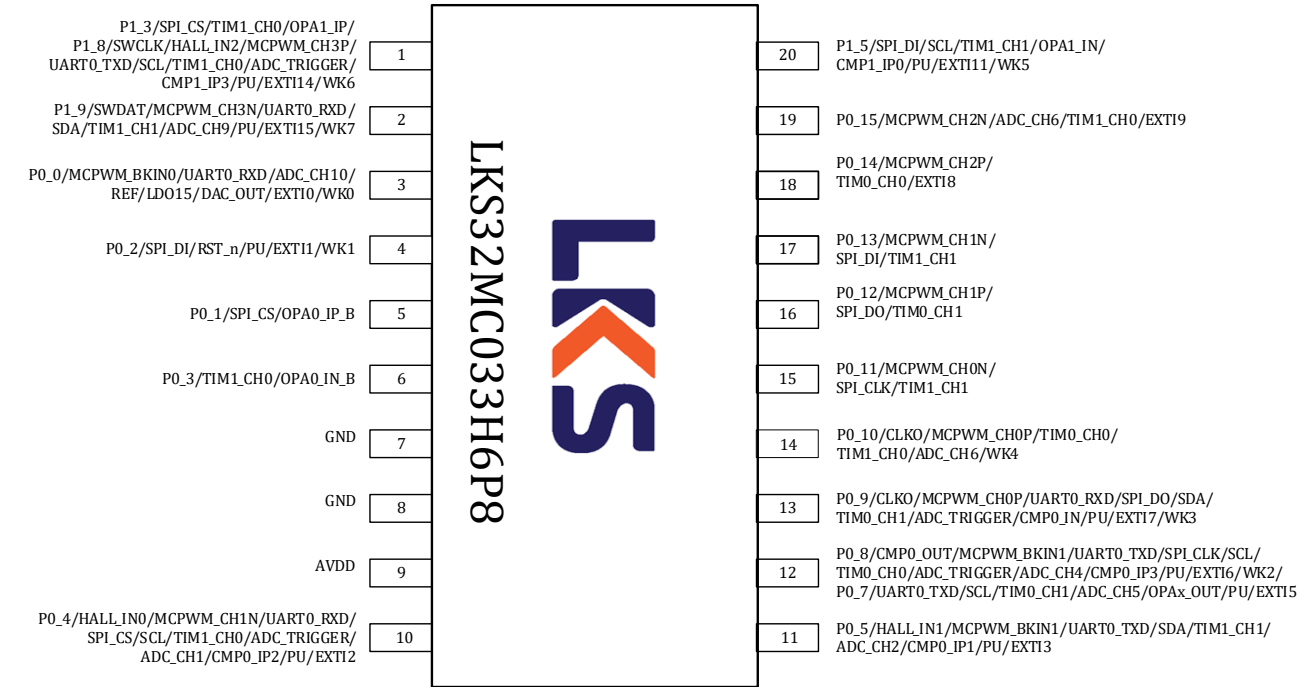
图 3-2 LKS32MC033H6P8 管脚分布图
