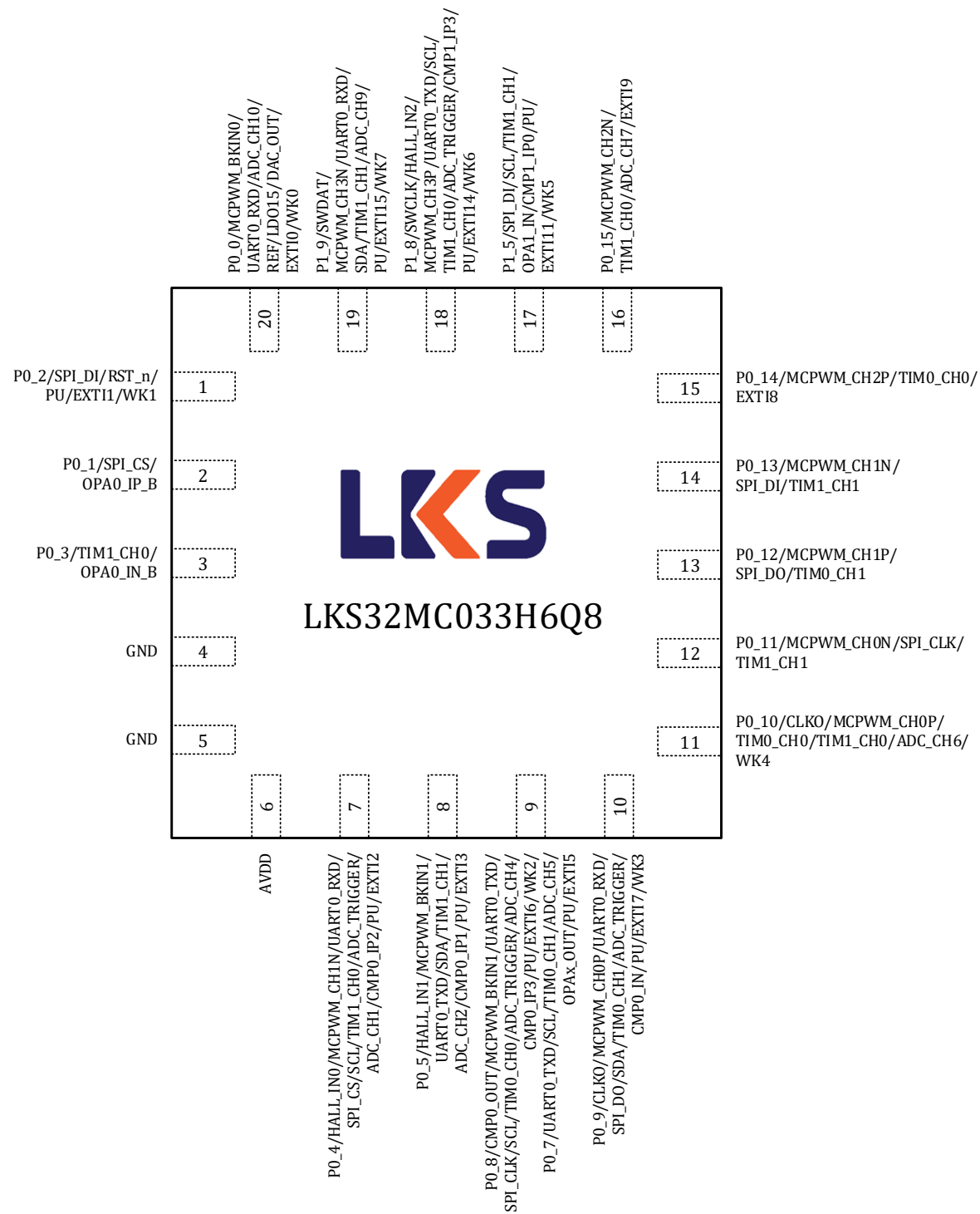
图 3-4 LKS32MC033H6Q8 管脚分布图
