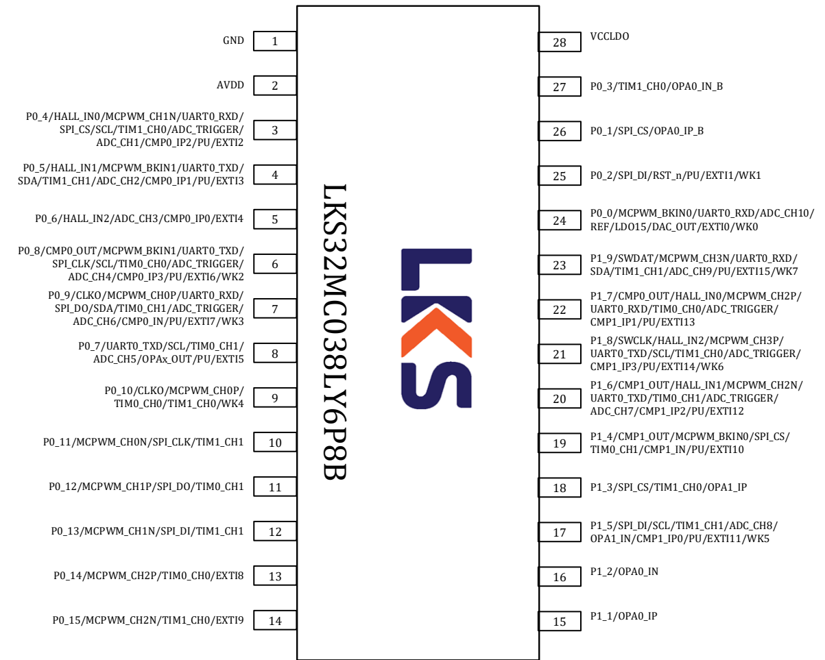
图 3-11 LKS32MC038LY6P8B/LKS32MC038LY6P8C 管脚分布图
