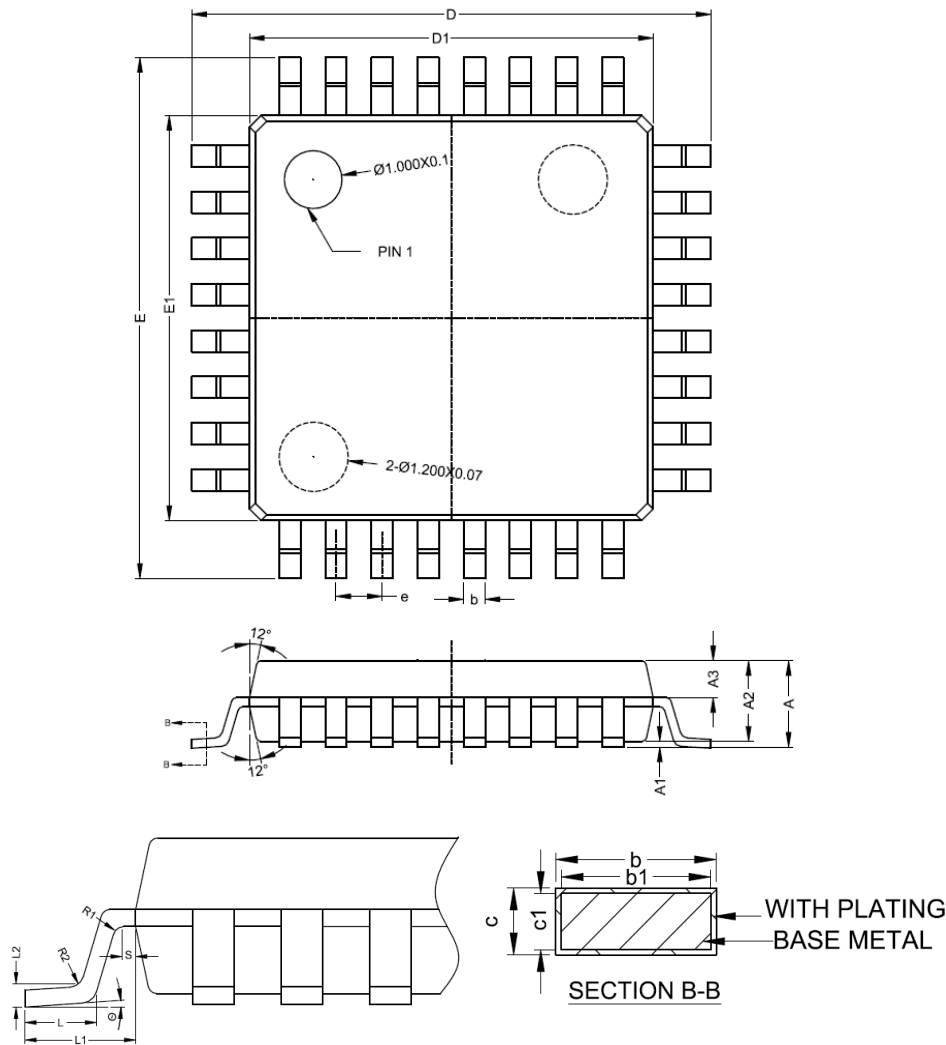
图 4-6 LKS32MC032LK6T8C 封装图示
