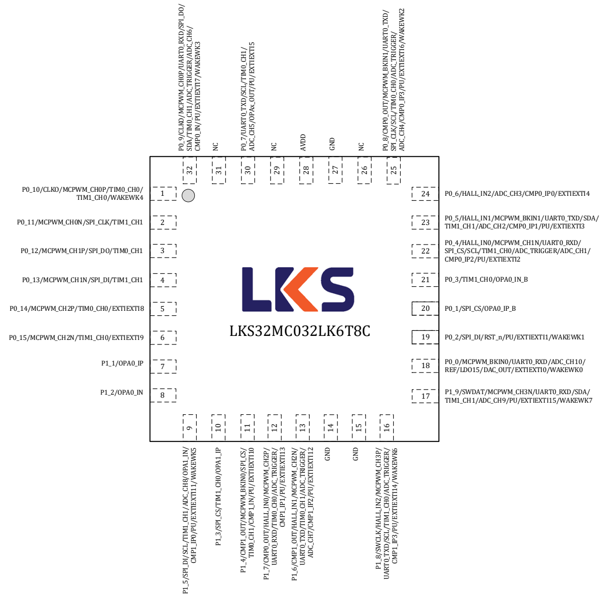
图 3-1 LKS32MC032LK6T8C 管脚分布图
