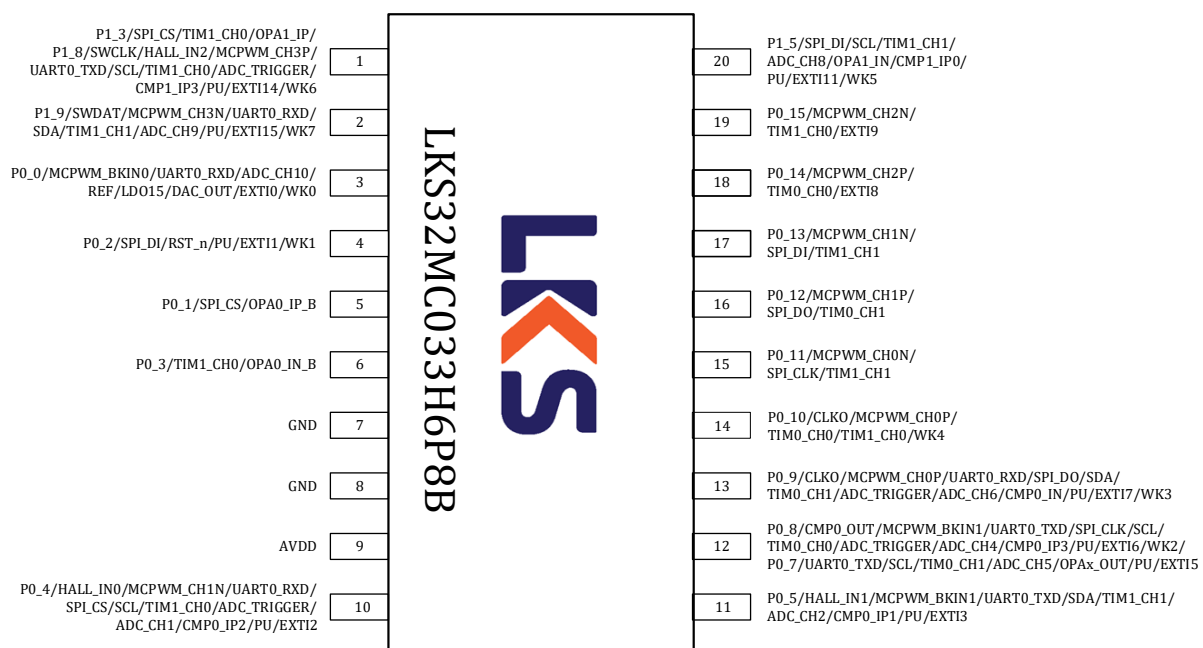
图 3-3 LKS32MC033H6P8B/LKS32MC033H6P8C 管脚分布图
