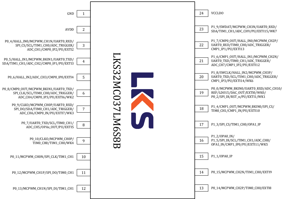
图 3-8 LKS32MC037LM6S8B/LKS32MC037LM6S8C 管脚分布图
