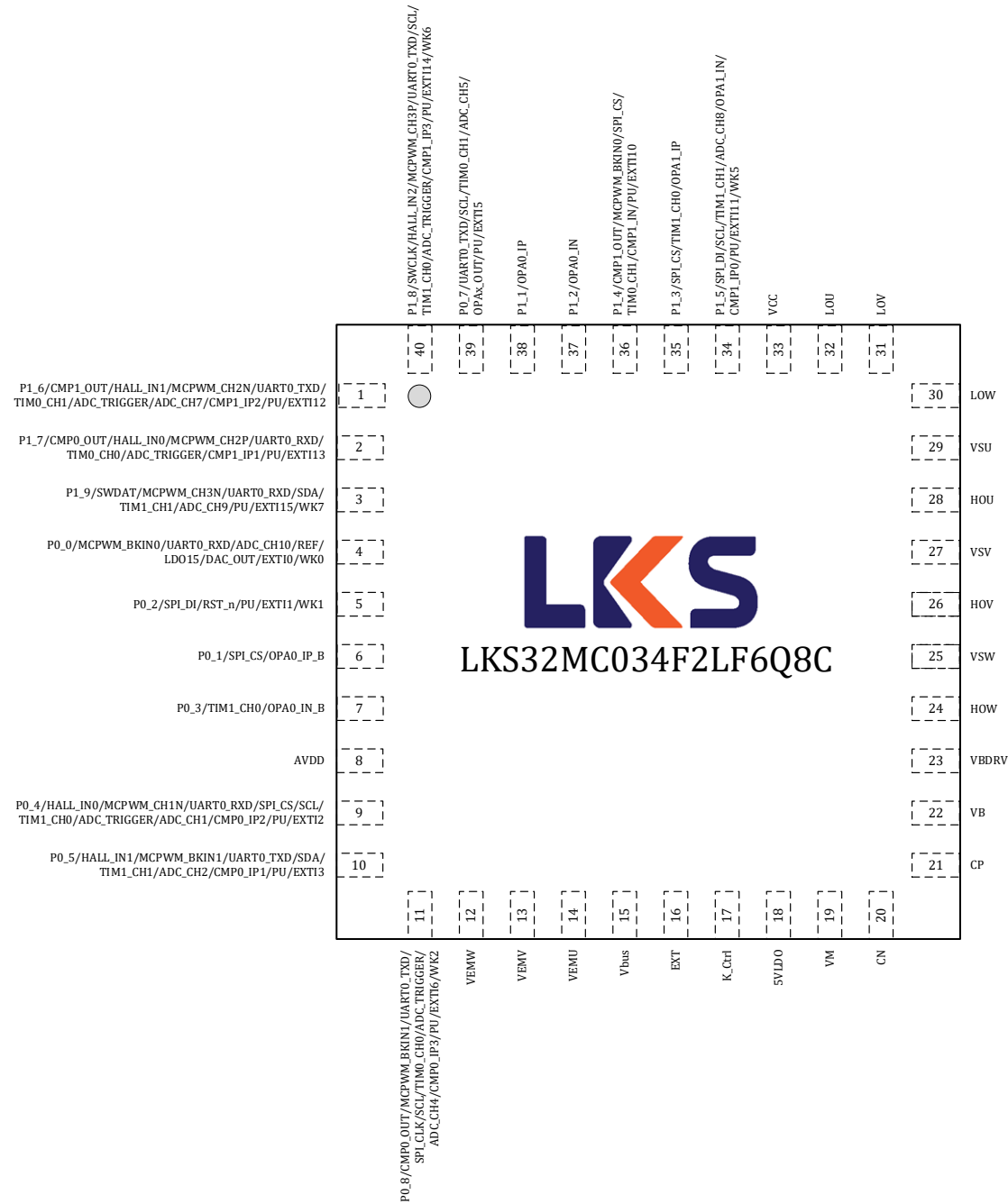
图 3-15 LKS32MC034F2LF6Q8C 管脚分布图
