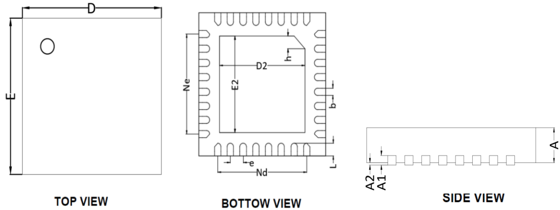
图 4-4 LKS32MC0342FLK6Q8C 封装图示
