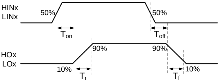
图 20-4 开关时序
