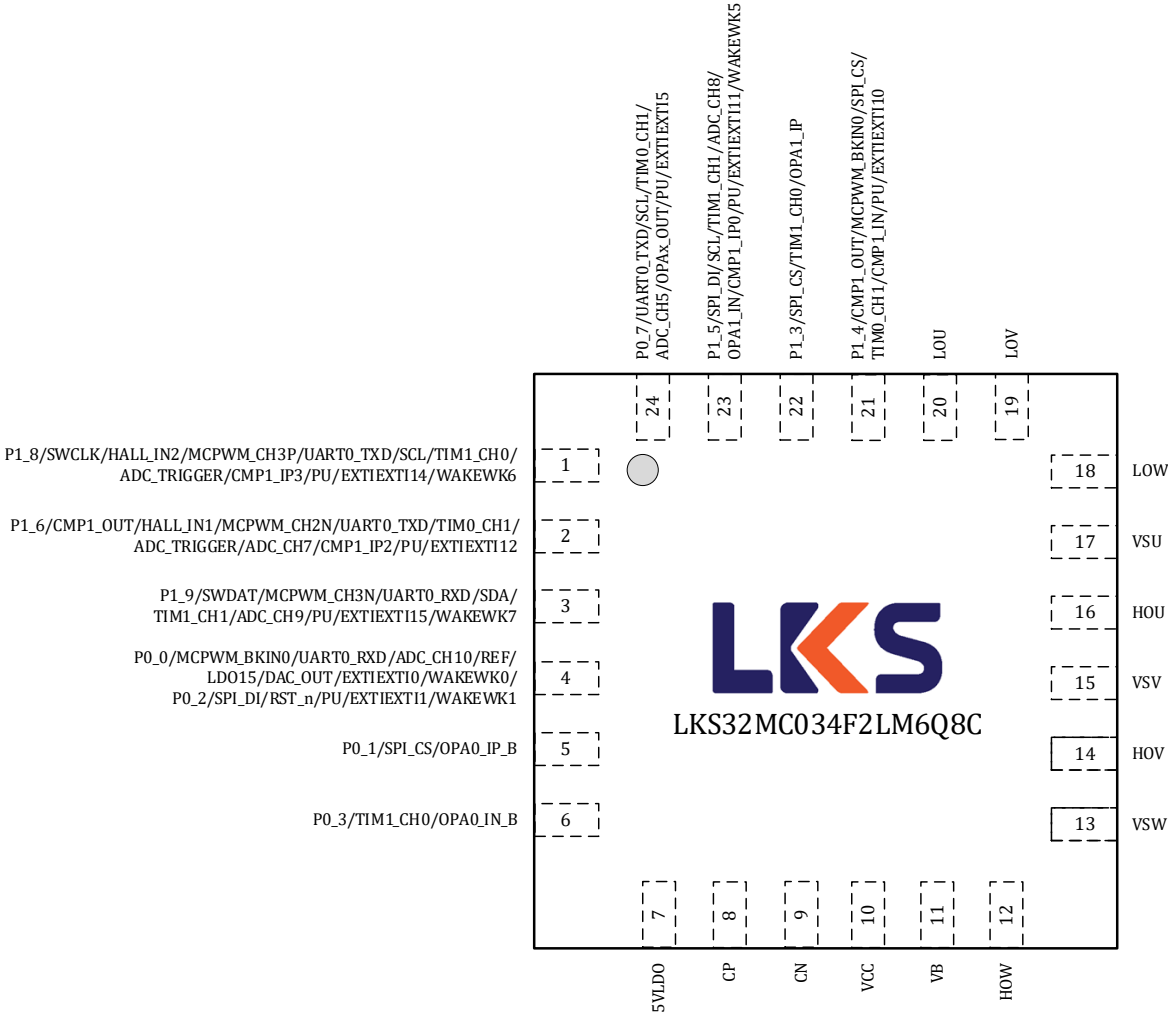
图 3-19 LKS32MC034F2LM6Q8C 管脚分布图
