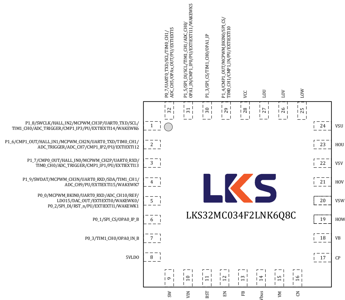
图 3-23 LKS32MC034F2LNK6Q8C 管脚分布图
