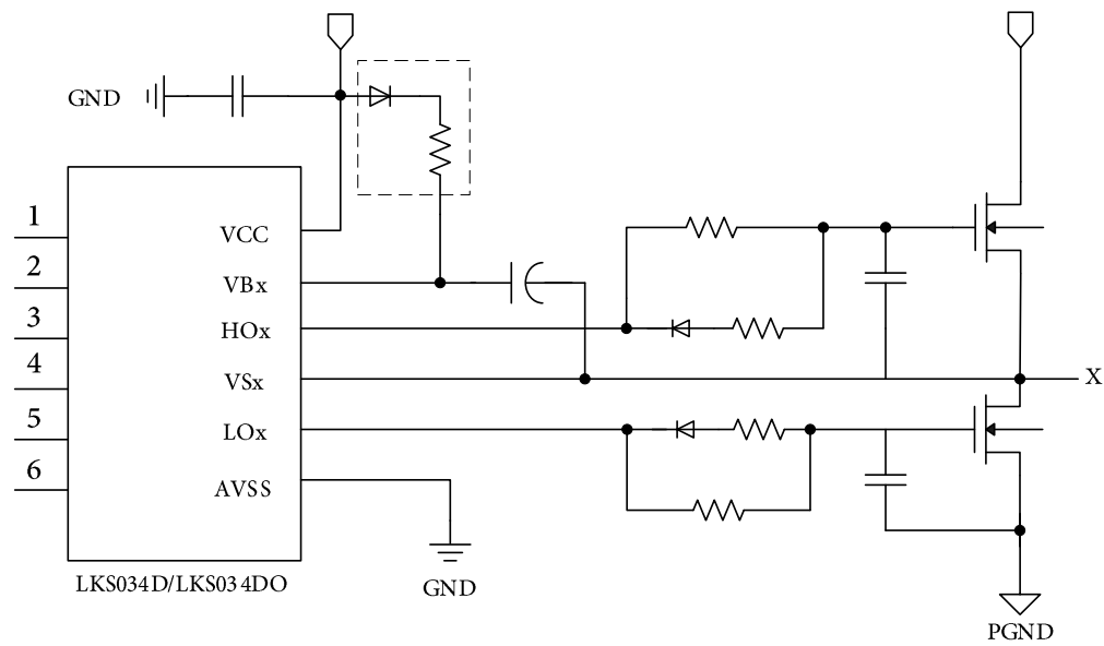
图 21-3 6N 型栅极驱动模块典型应用图 LKS034D(O)
