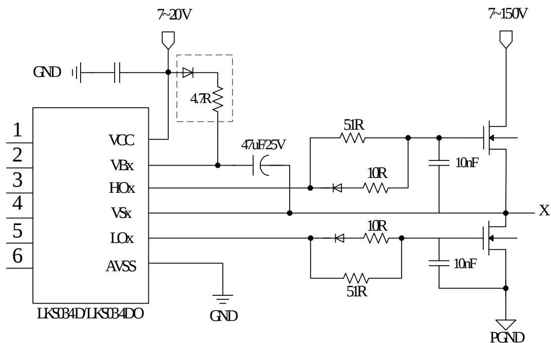
图 21-3 6N 型栅极驱动模块典型应用图 LKS034D(0)
