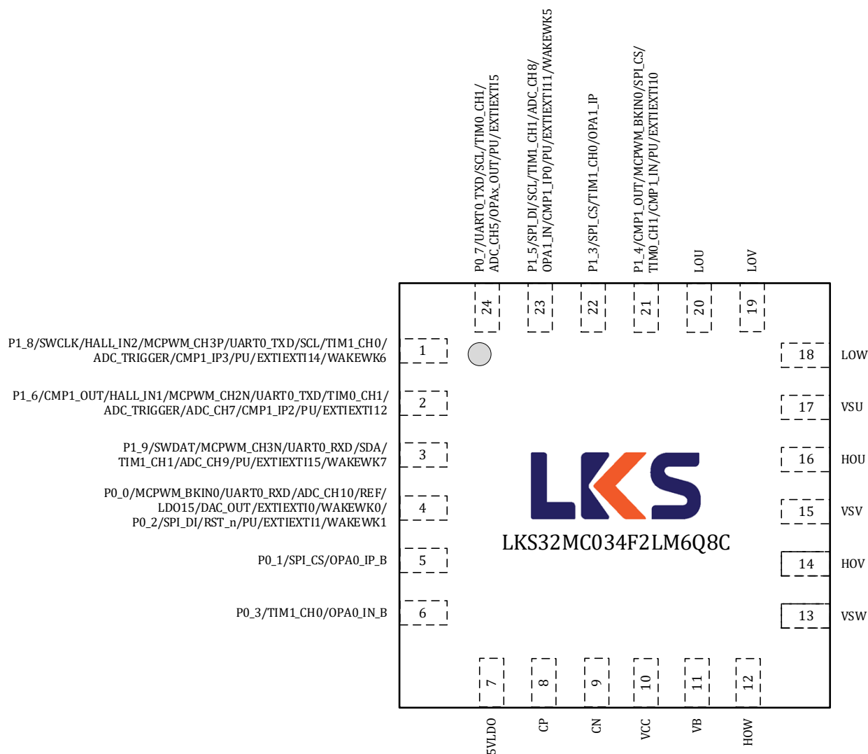
图 3-19 LKS32MC034F2LM6Q8C 管脚分布图
