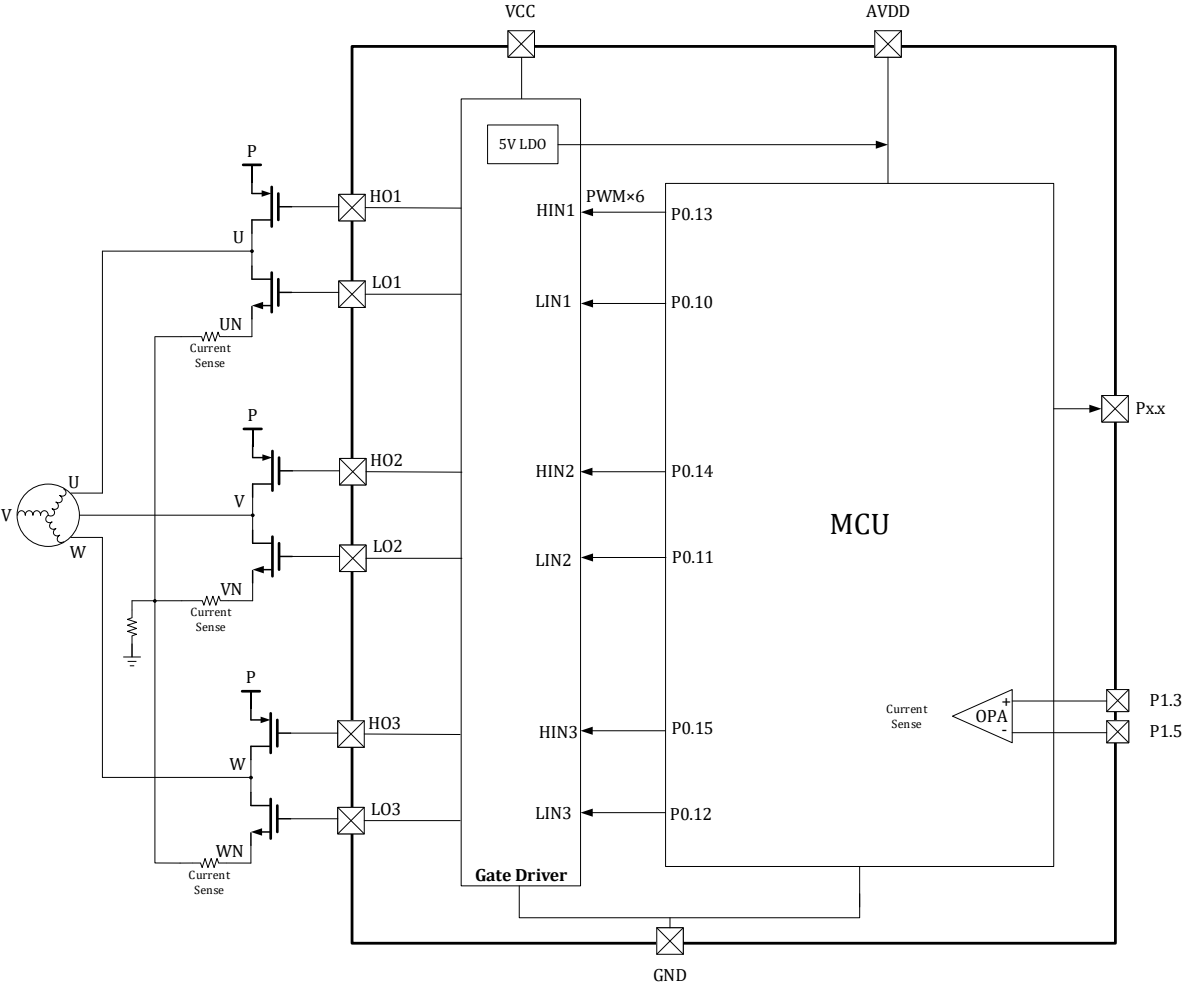
图 3-4 LKS32MC035DL6S8 预驱连接示意图
