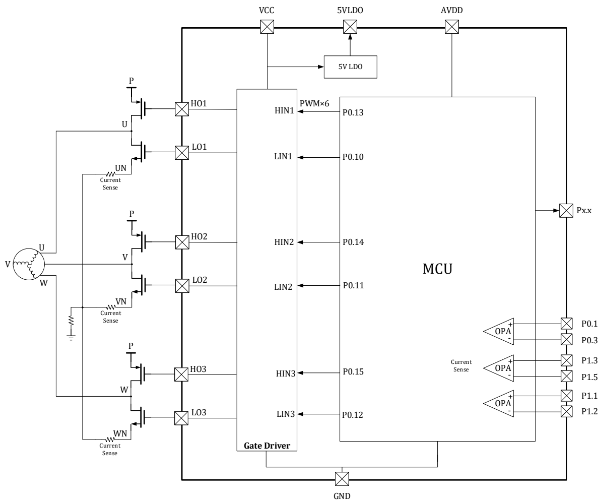
图 3-20 LKS32MC039DK6Q8B(C)预驱连接示意图
