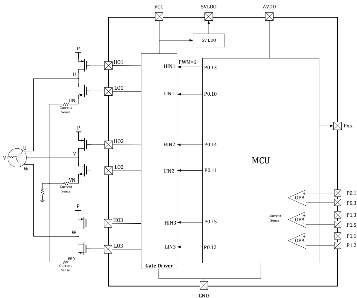
图 3-20 LKS32MC039D2K6Q8C 预驱连接示意图
