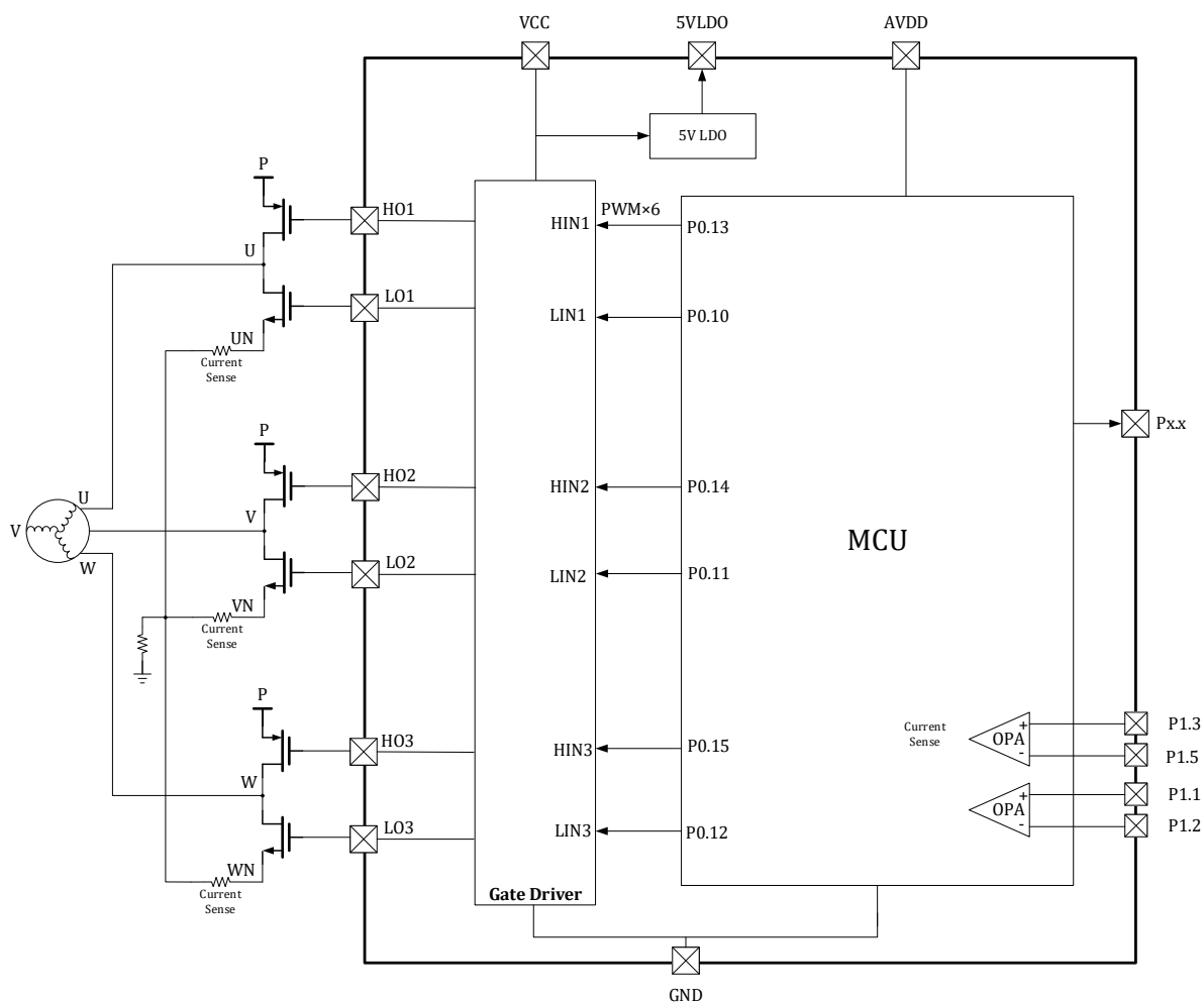
图 3-16 LKS32MC037QM6Q8 预驱连接示意图
