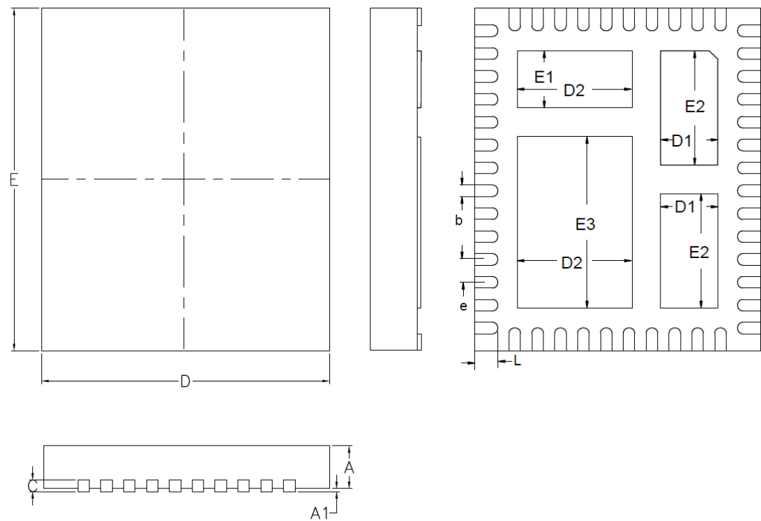
图 4-1 LKS32MC031PC6Q8C 封装图示
