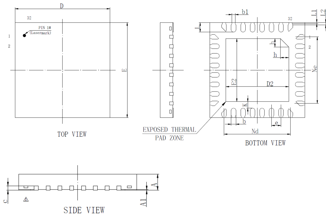
图 4-6 LKS32MC039PL3K6Q8C 封装图示
