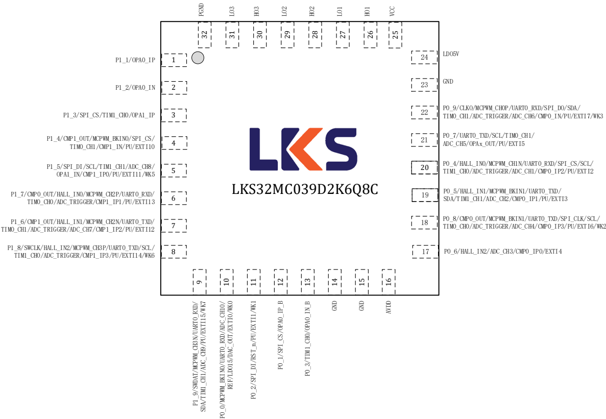
图 3-19 LKS32MC039D2K6Q8C 管脚分布图
