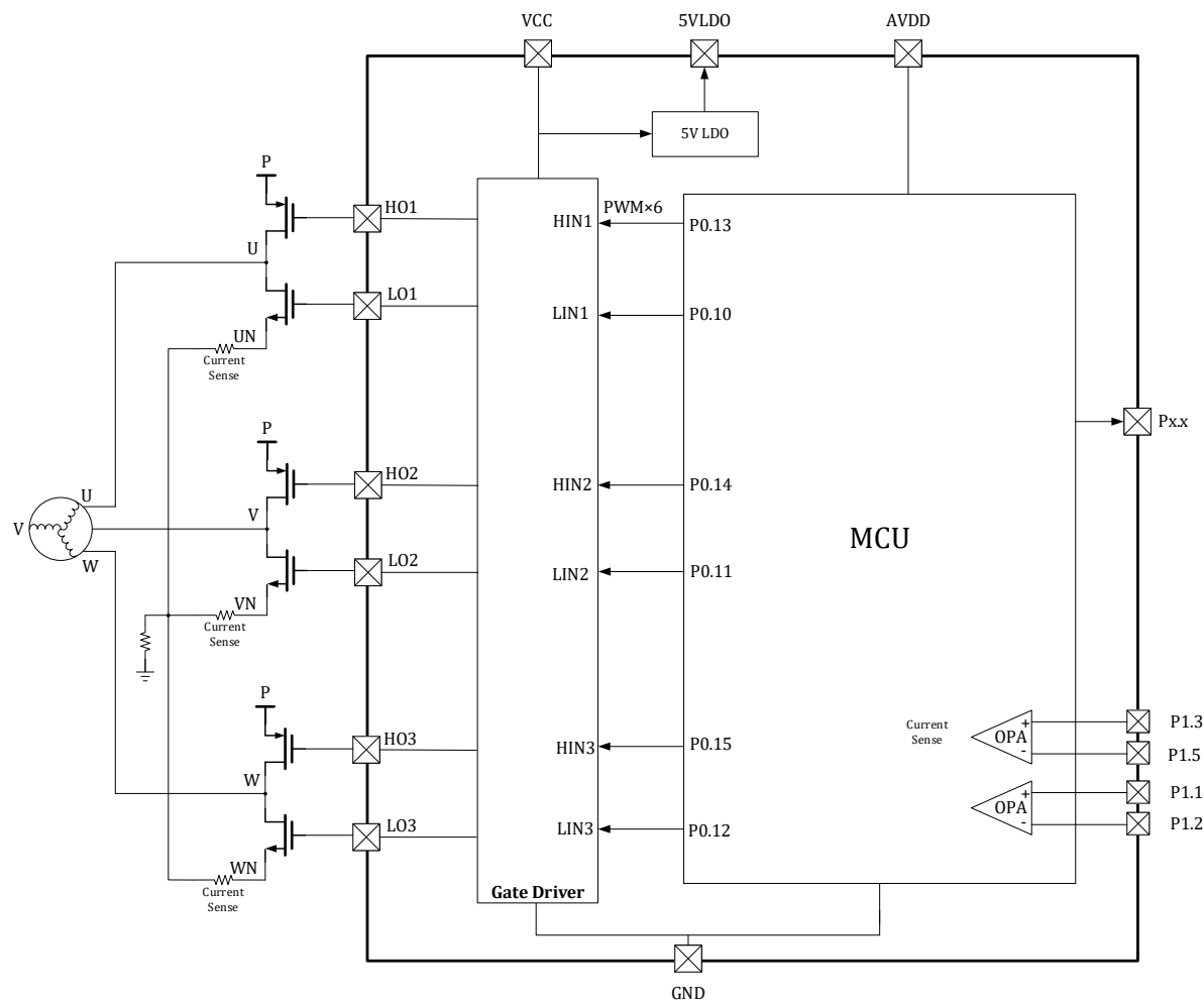
图 3-12 LKS32MC037EM6S8C 预驱连接示意图
