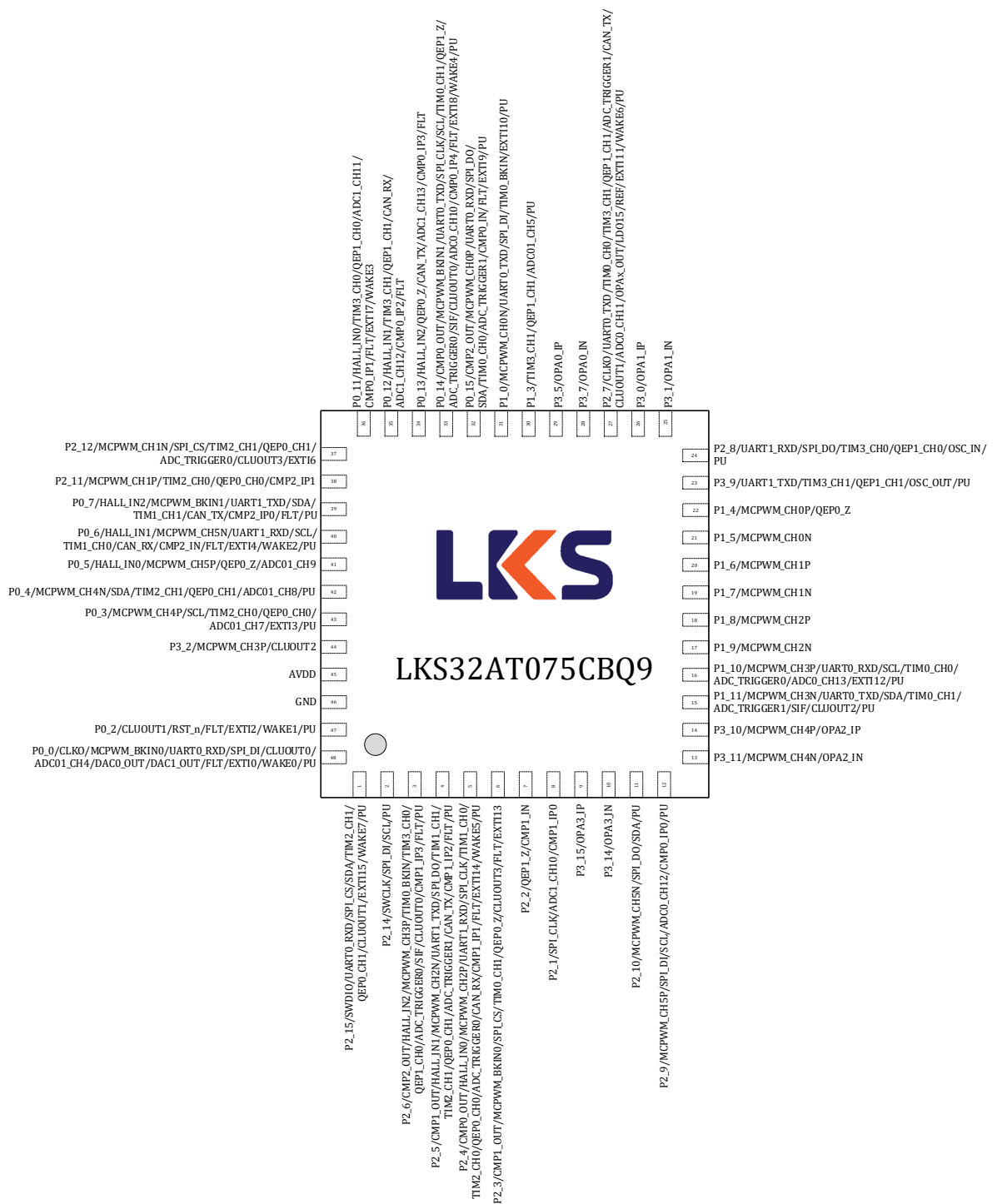
图 2-1 LKS32AT075CBQ9 管脚分布图
