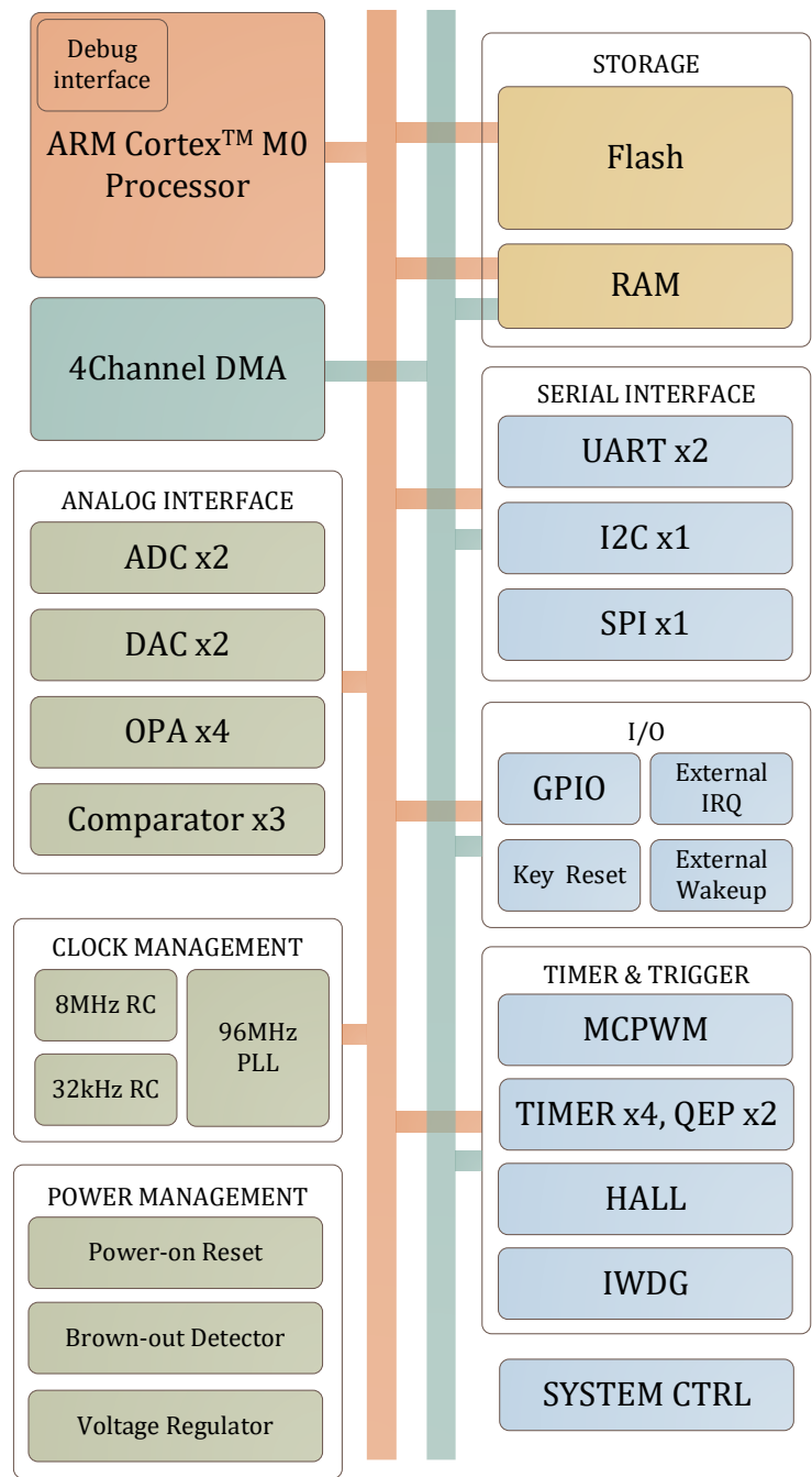
图 2-3 LKS32AT075CBQ9 系统资源框图
