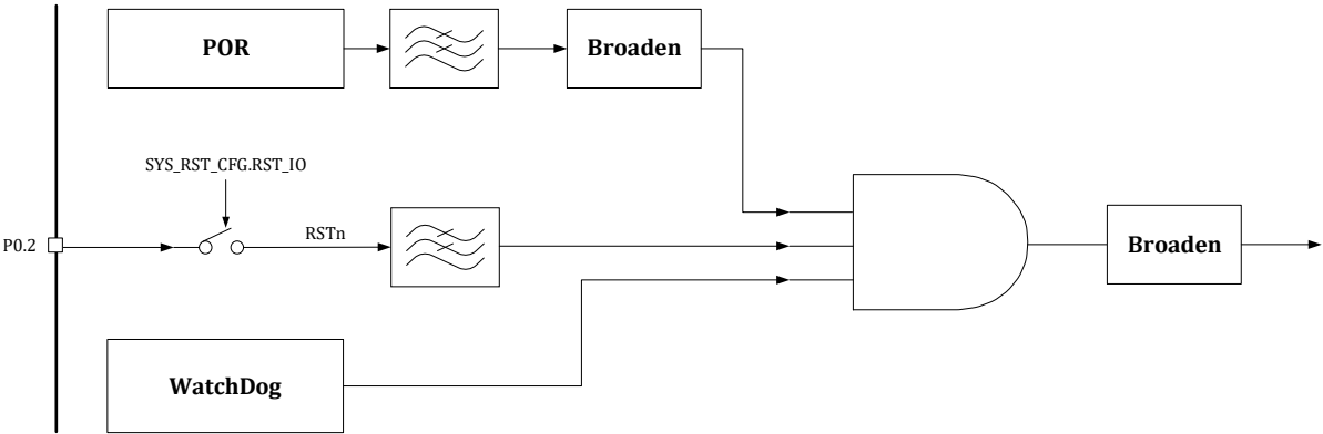
图 6-2 复位架构
