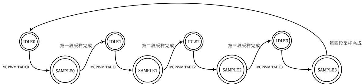
图 12-5 ADC 四段采样状态转移图
