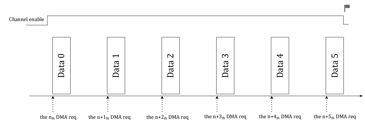
图 17-3 RMODE=1 DMA 传输情况
