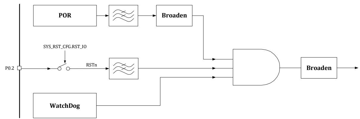
图 6-2 复位架构
