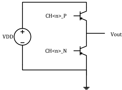
图 14-11MCPWM IO 控制示意图
