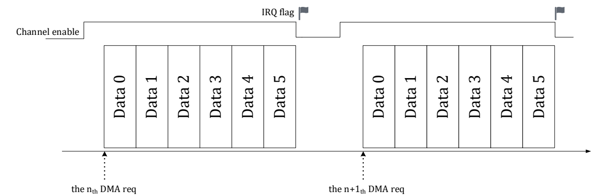
图 17-2 RMODE=0 DMA 传输情况
