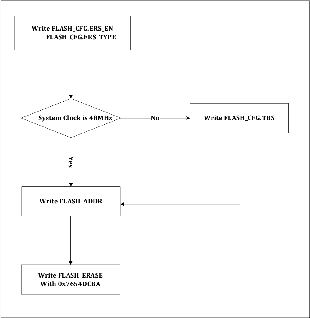
图 7-6 FLASH 模块擦除操作流程图
