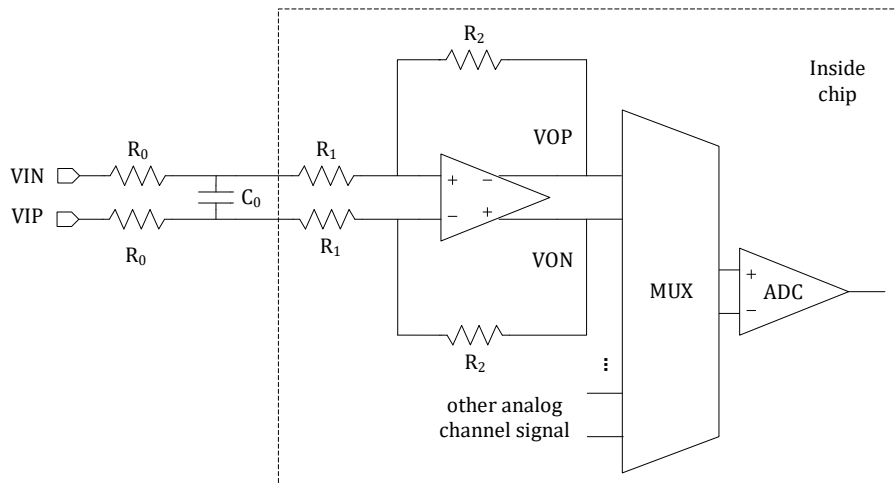
图 5-2 放大器框图
