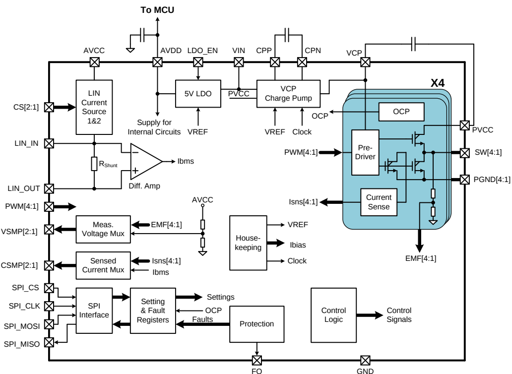
图 21-1 IPM 模块结构框图
