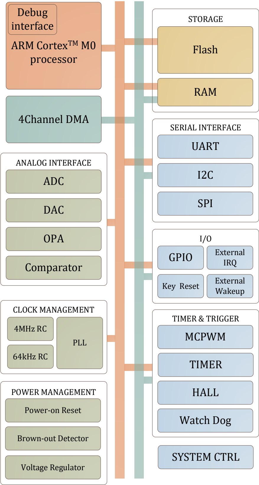
图 2-1 LKS32AT03x 系统框图
