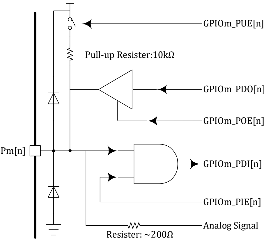
图 15-1 GPIO 功能框图
