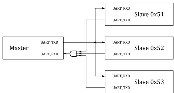
图 16-3 UART 多机通讯示例
